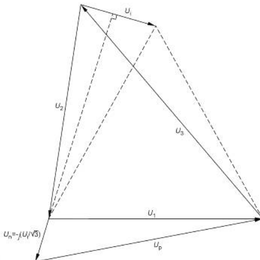
Рисунок А.1 — Векторная диаграмма
