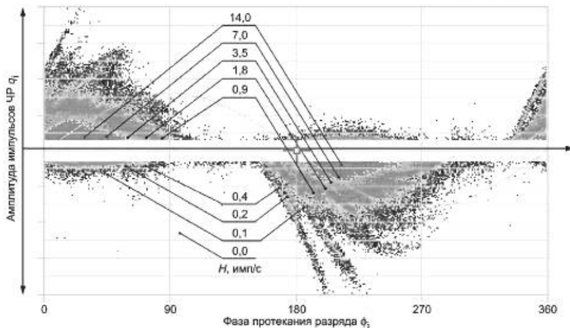
Рисунок 4 — Пример \varphi - q - n диаграммы рассеяния импульсов ЧР на объекте, представленном на рисунке 5b.
