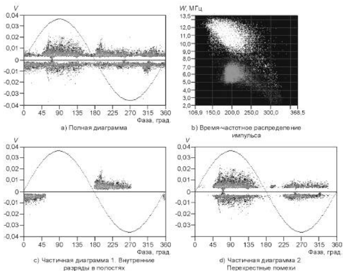
Рисунок D.5 — Пример выделения перекрестных помех
