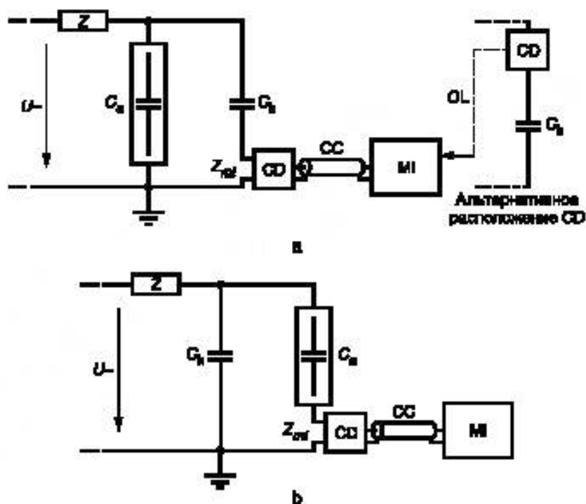
а — соединительное звено последовательно с соединительным конденсатором; б — соединительное звено последовательно с испытуемым объектом; U — высоковольтный источник; Z_{\text{вх}} — входное сопротивление измерительной системы; CC — соединительный кабель; OL — оптическая линия связи; C_d — испытуемый объект; C_k — соединительным конденсатором; CD — соединительное звено; MI — измерительный прибор; Z — фильтр
