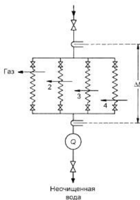
Рисунок 2 – Параллельное соединение охладителей
