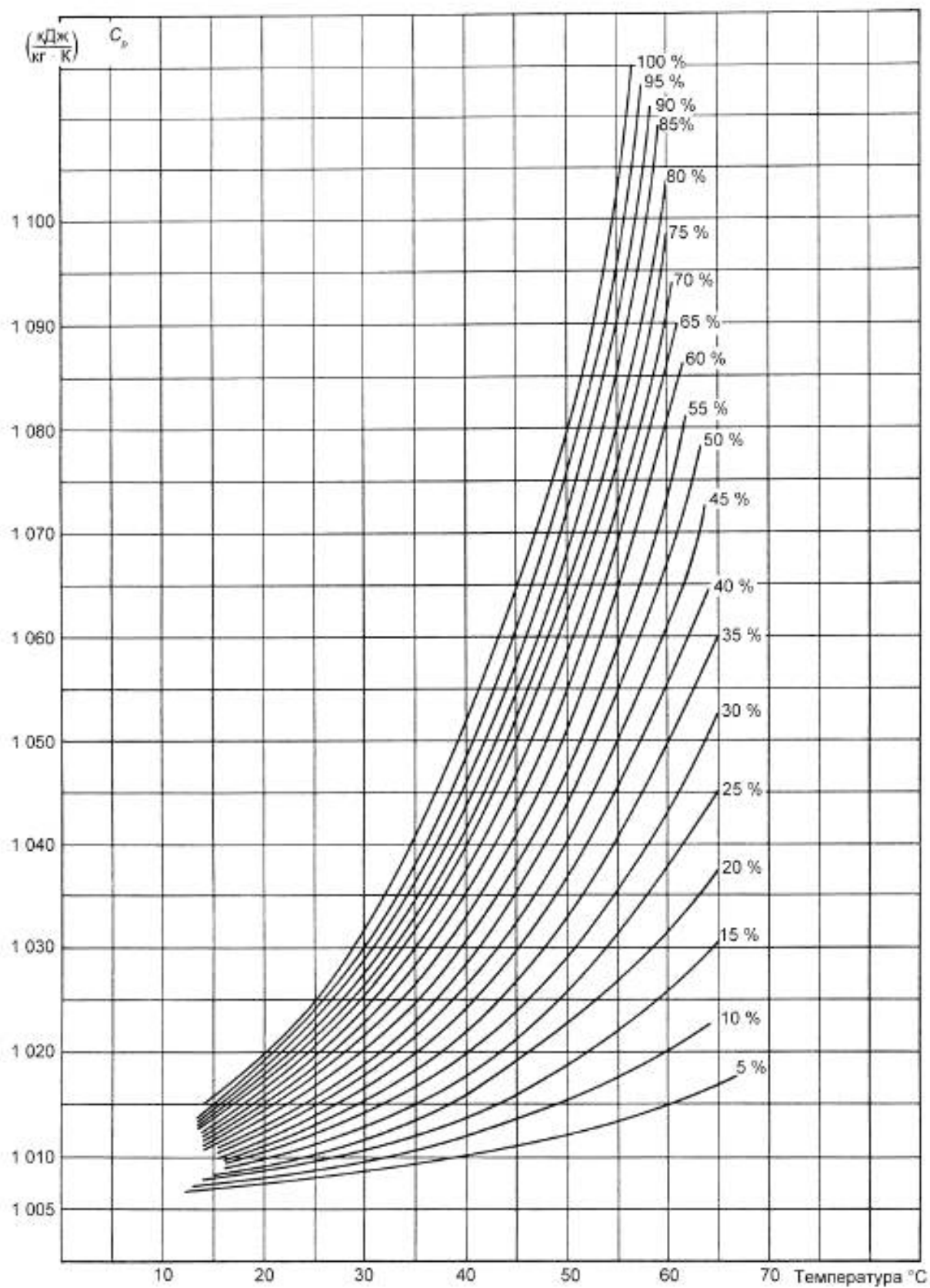
Рисунок В – Удельная теплоемкость c_p воздуха для различных значений влажности и температуры
