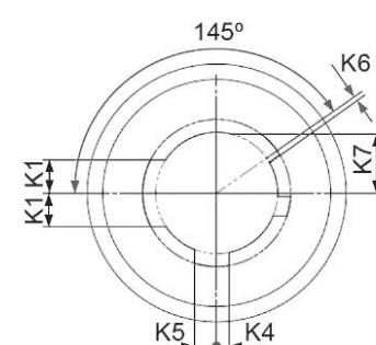
Тип K6
