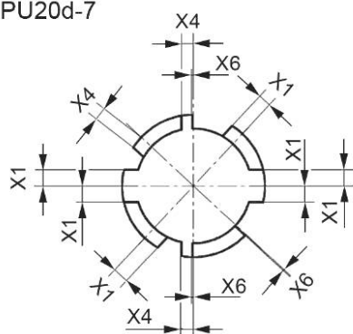
PU20d-7
