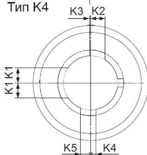
Тип K4
