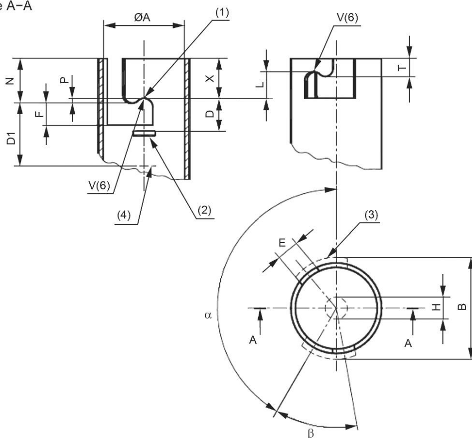
Сечение А-А
