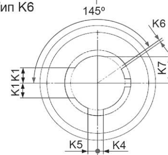
Тип K6
