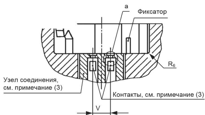
Сечение I-I
