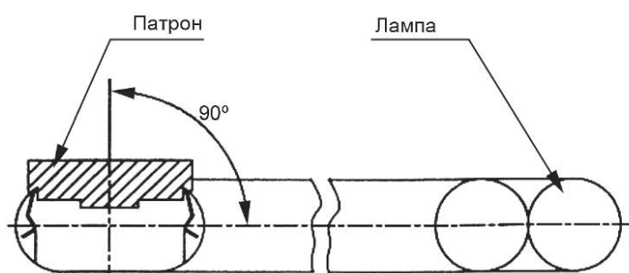
Монтажное положение лампы и патрона
