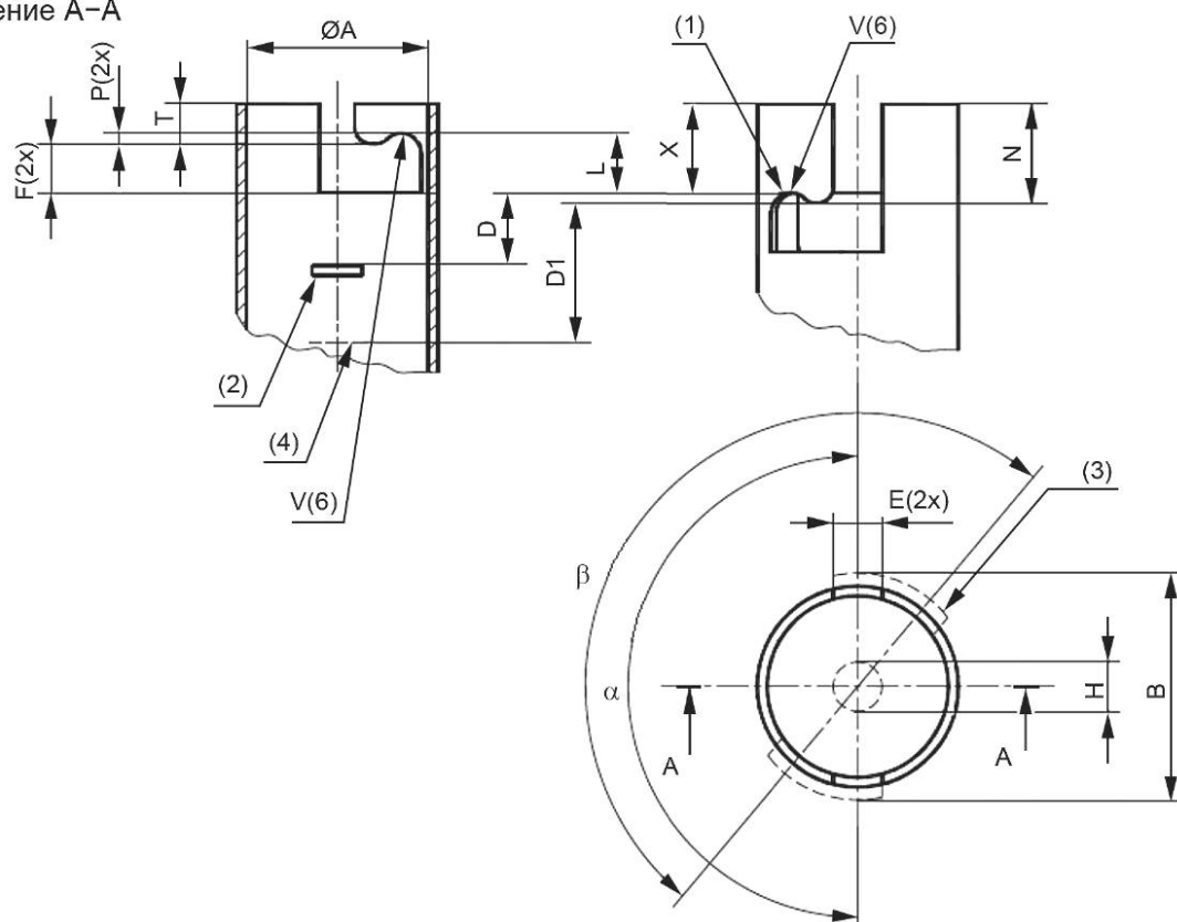
Сечение А-А
