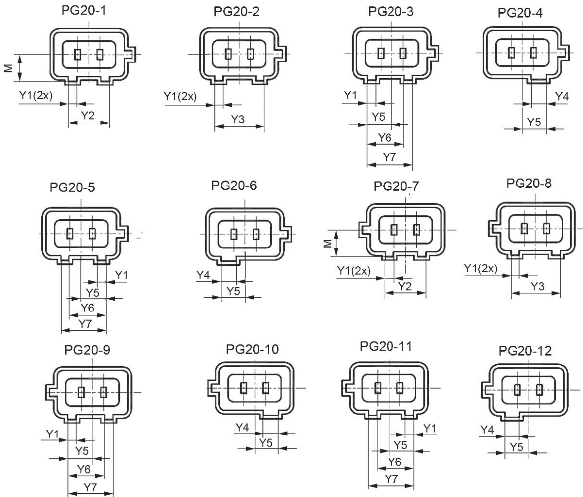
Фиксаторы соединителя PG20
