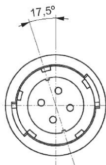
GR14q-1
