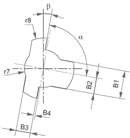
Монтажное отверстие
