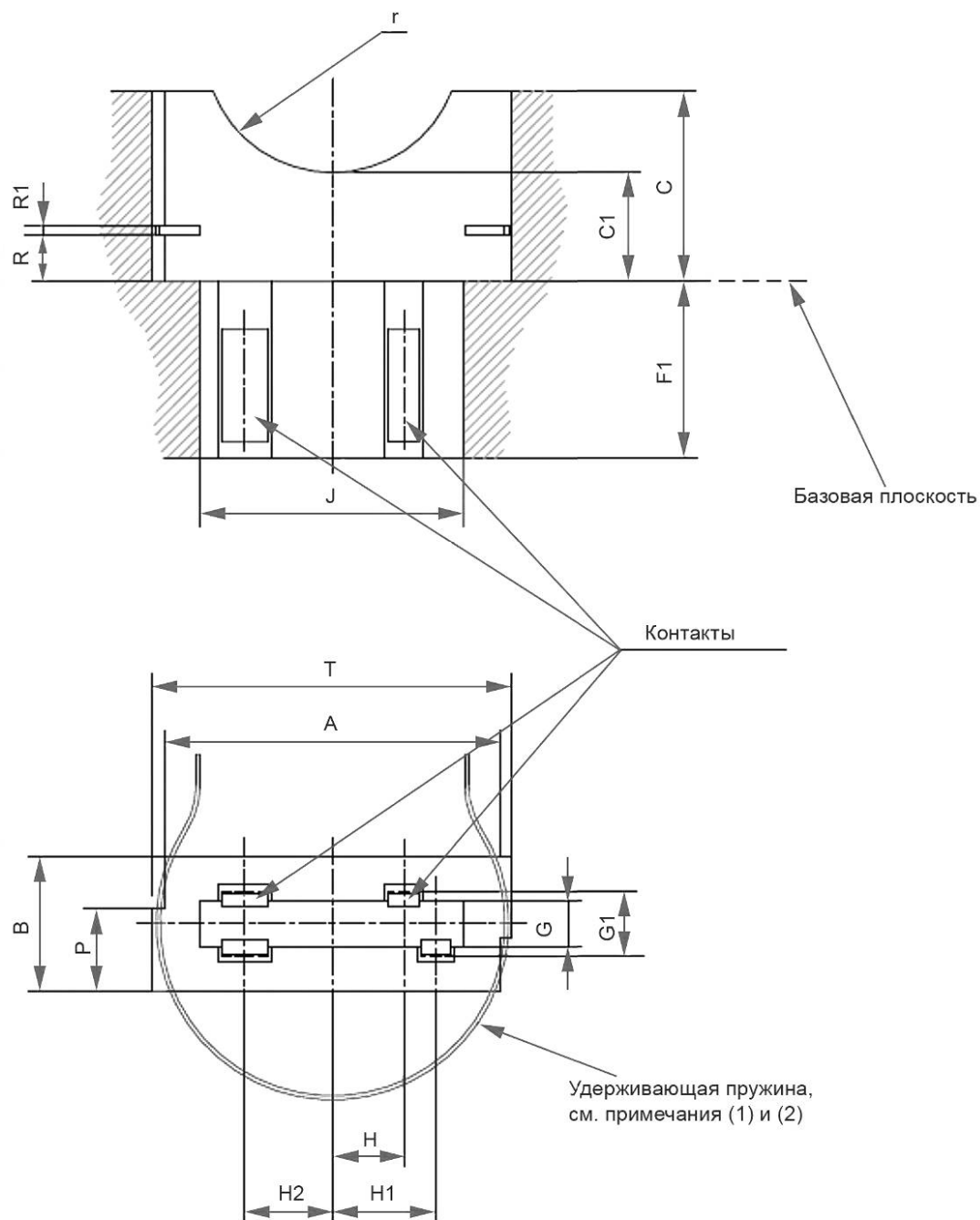
Патрон типа В
