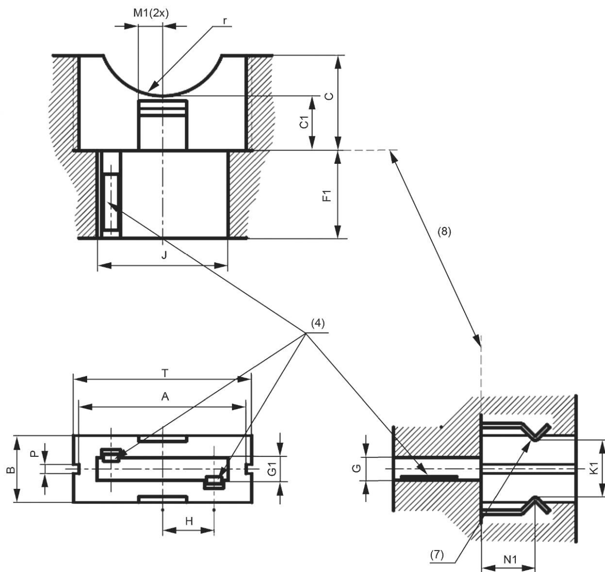
Патрон типа А
