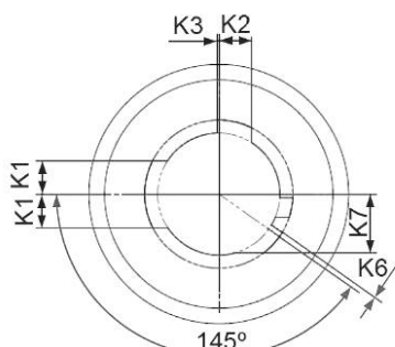
Тип K5
