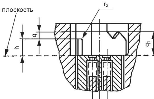
Сечение II-II
