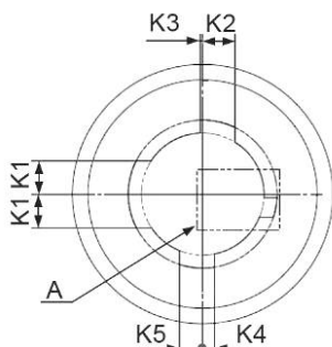
Тип K4
