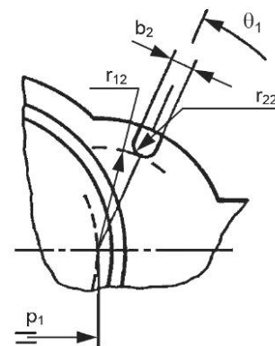
Сечение II-II
