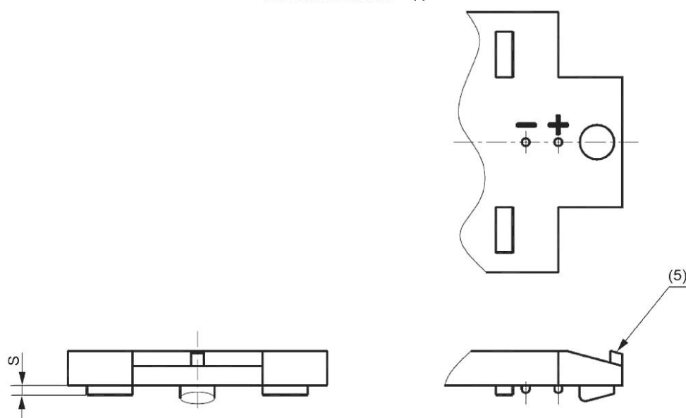
Тип В — Штепсельный соединитель
