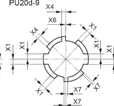
PU20d-9
