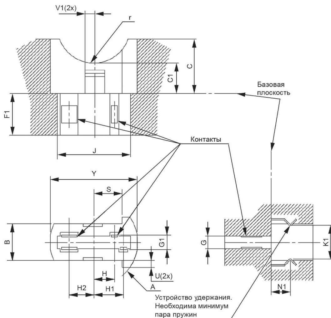
Форма базового паза
