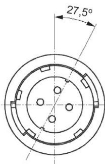
GR14q-2
