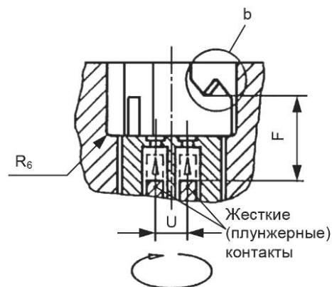
Сечение III-III
