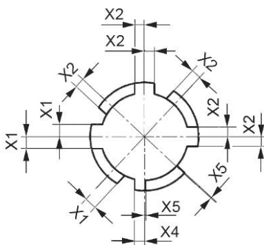
PU20d-5
