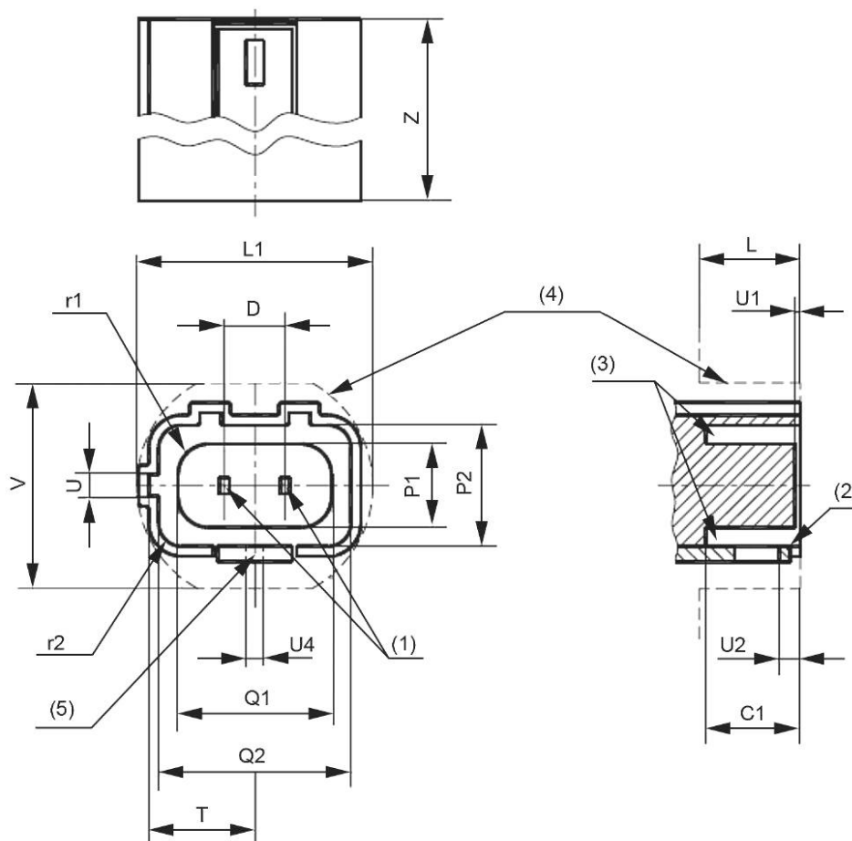
Соединитель PG20
