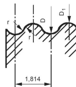
Деталь резьбы Правая резьба
