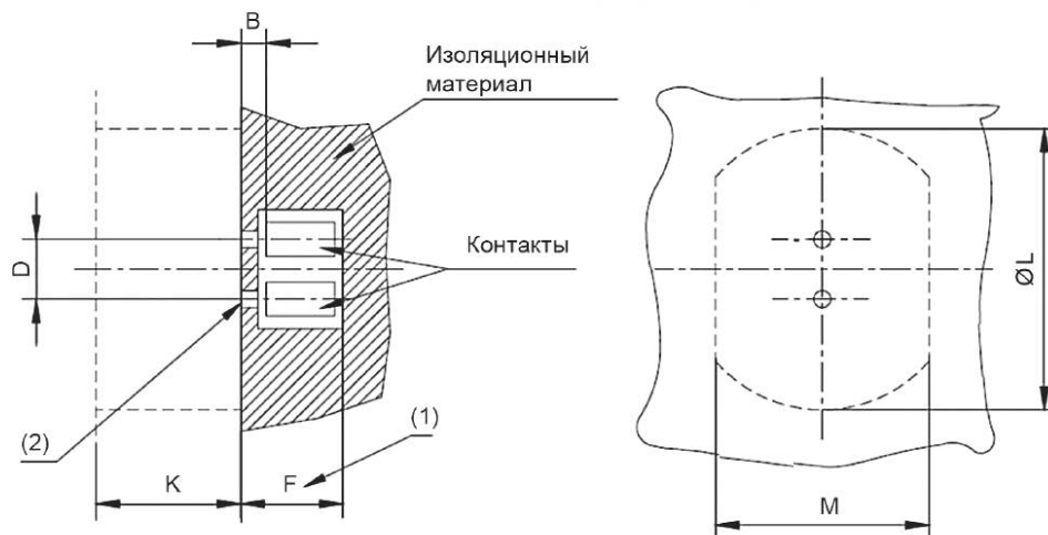
Рисунок 1 — Соединитель
