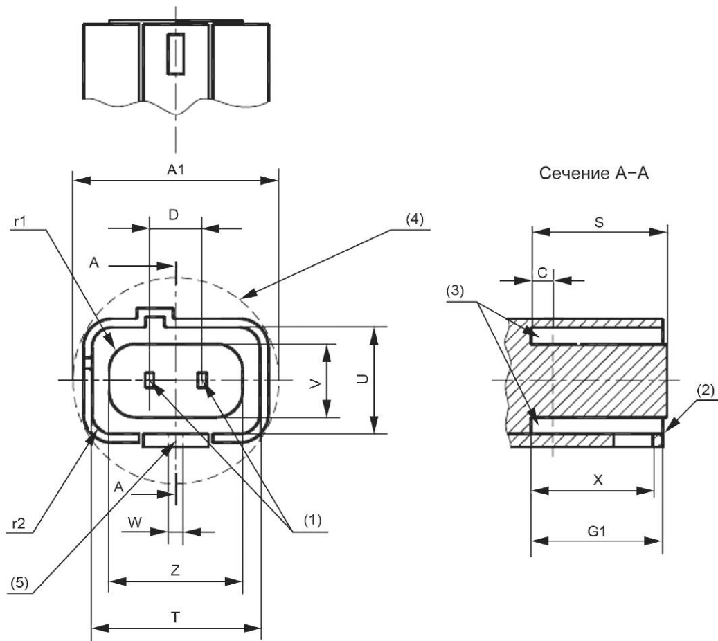
Соединитель PG18.5d
