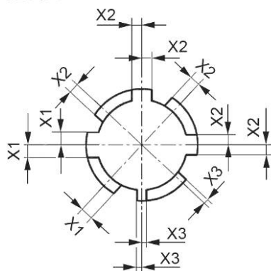
PU20d-7
