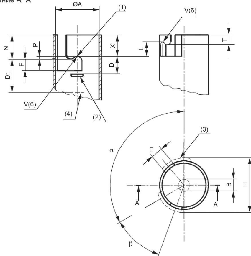
Сечение А-А
