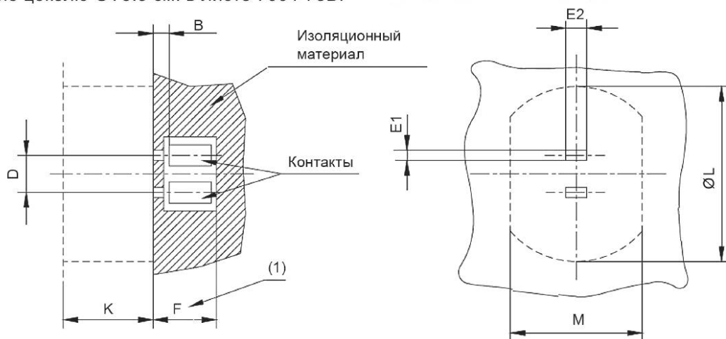
Рисунок 1 — Соединитель
