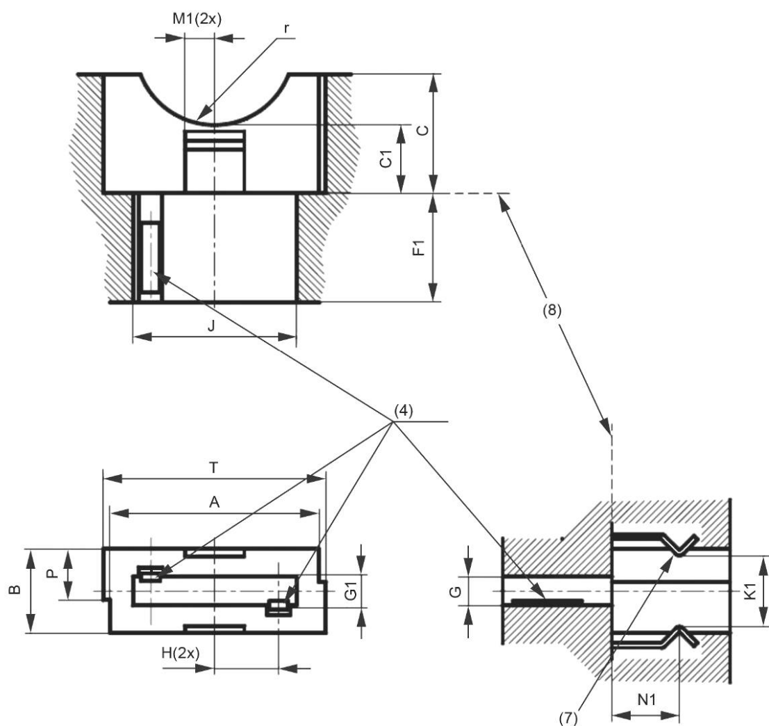
Патрон типа А
