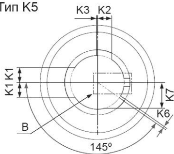
Рисунок 2, лист 1 — Размеры фиксаторов
