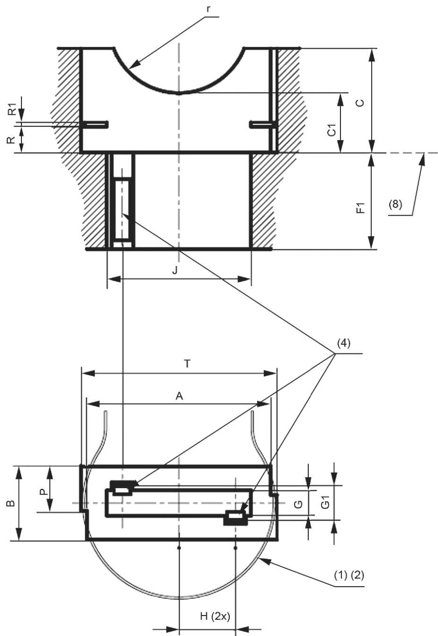
Патрон типа В
