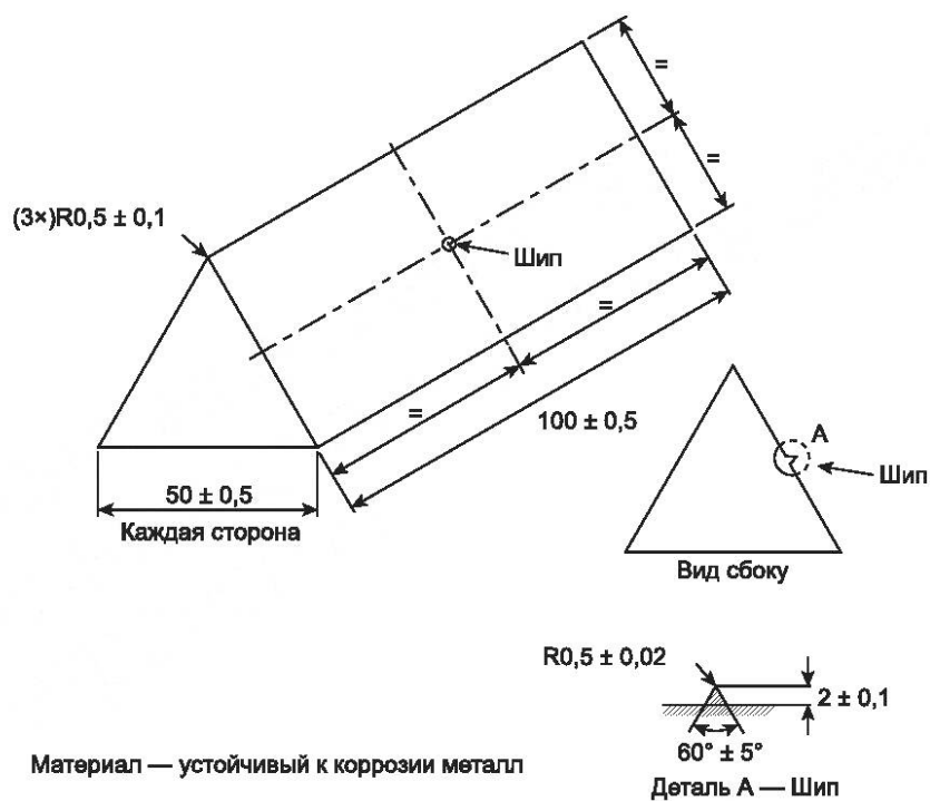
Рисунок 14 — Оправка
