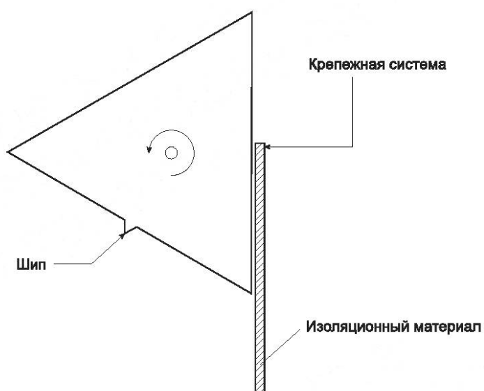
Рисунок 15 — Начальное положение оправки
