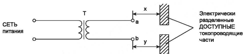
Рисунок 1 — Схема испытательной цепи для условий неисправности
