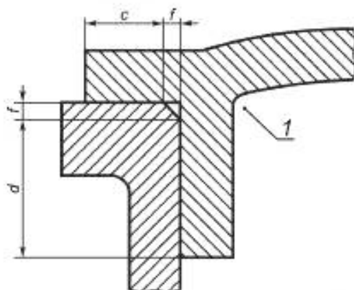
Рисунок 2а — Цилиндрическая часть
