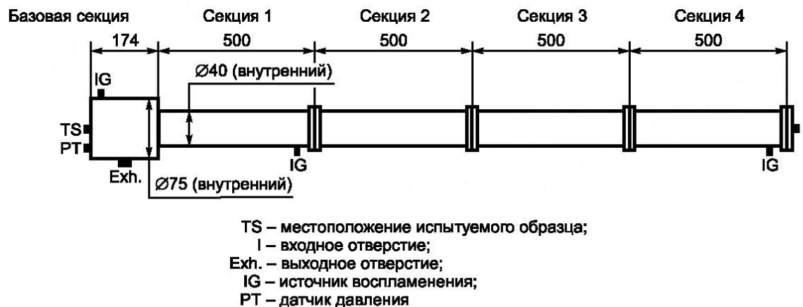
Рисунок 21 — Установка для испытаний дыхательных и дренажных устройств
