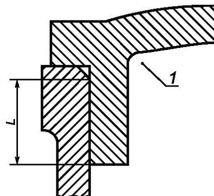
Рисунок 2б — Только Цилиндрическая часть
