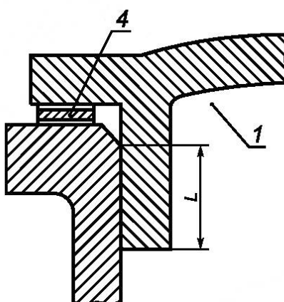
Рисунок 15 — Иллюстрация требований к прокладкам (пример 6)
