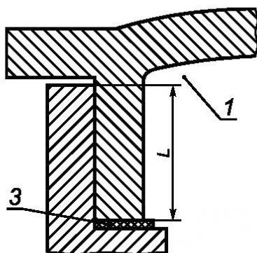
Рисунок 12 — Иллюстрация требований к прокладкам (пример 3)
