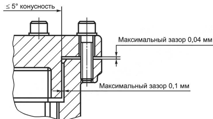
Рисунок J.3 — Конический компоновочный узел между крышкой и корпусом
