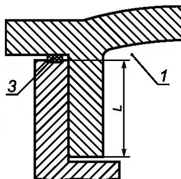
Рисунок 13 — Иллюстрация требований к прокладкам (пример 4)
