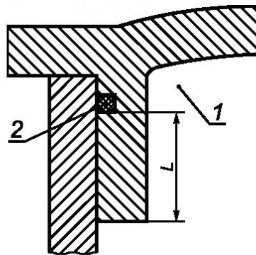
Рисунок 11 — Иллюстрация требований к прокладкам (пример 2)
