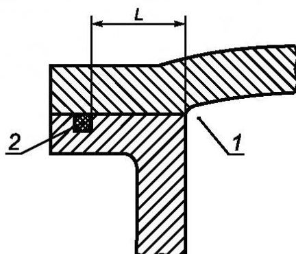
Рисунок 14 — Иллюстрация требований к прокладкам (пример 5)
