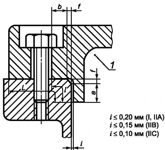
Рисунок 6 — Отверстия на поверхностях плоскоцилиндрических соединений (пример 1)
