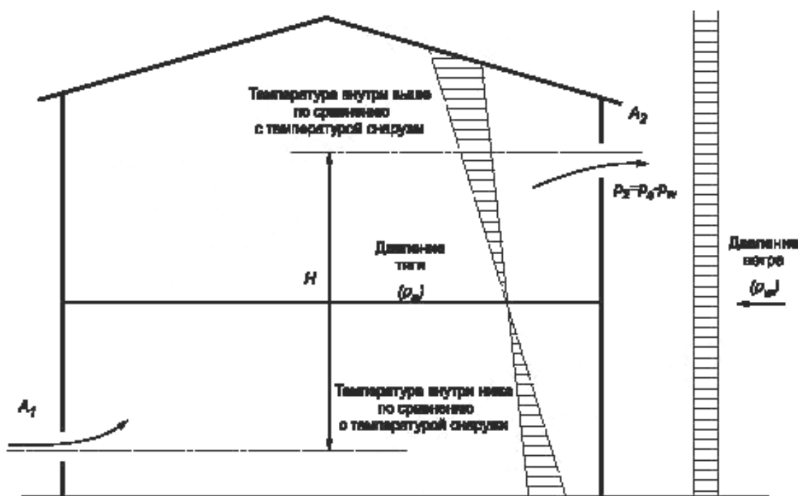
Рисунок С.1 — Пример противодействующих движущих сил вентиляционных потоков
