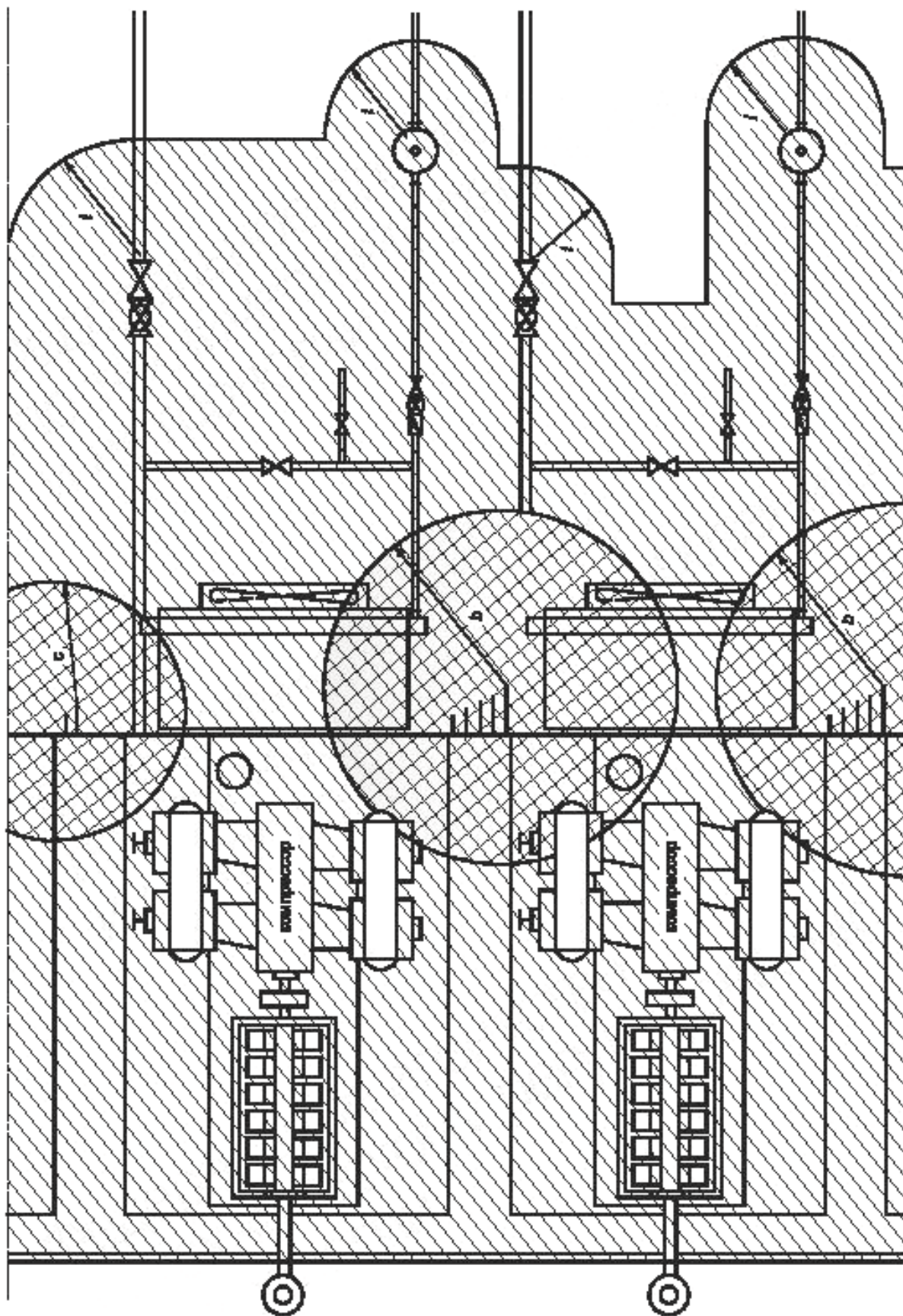
Рисунок D. 1а — Пример классификации зон для компрессора, работающего на природном газе
