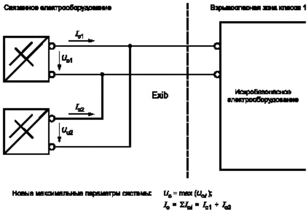
Рисунок 1.2 — Параллельное соединение. Суммирование значений тока
