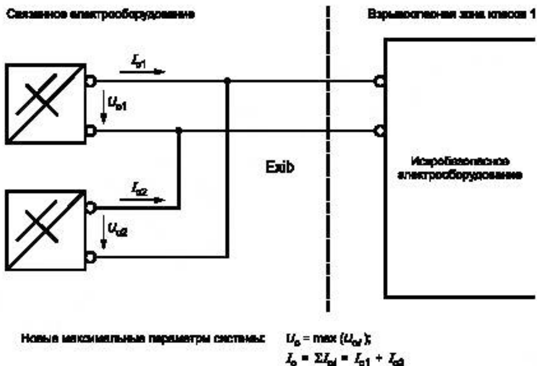
Рисунок I.2 — Параллельное соединение. Суммирование значений тока
