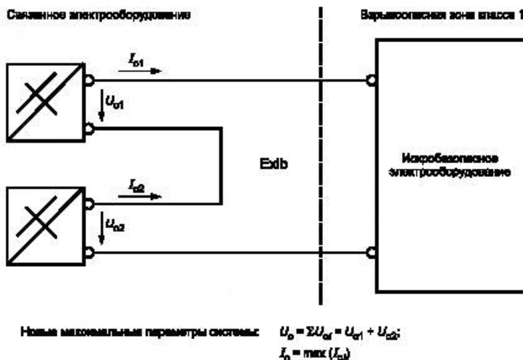
Рисунок I.1 — Последовательное соединение.
