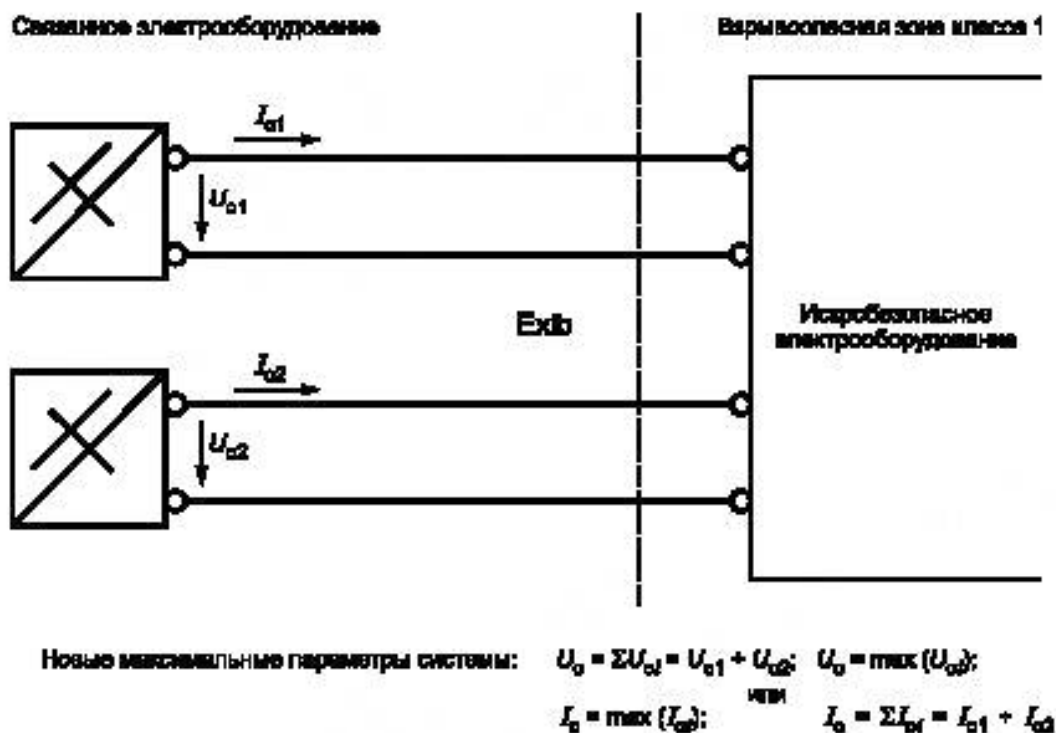
Рисунок I.3 — Последовательные и параллельные соединения.
