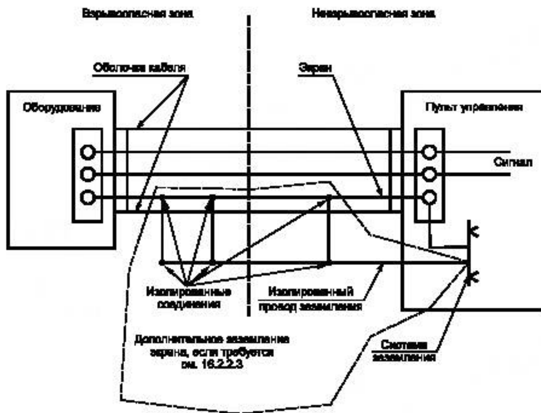
Рисунок 2 — Заземление проводящих экранов
