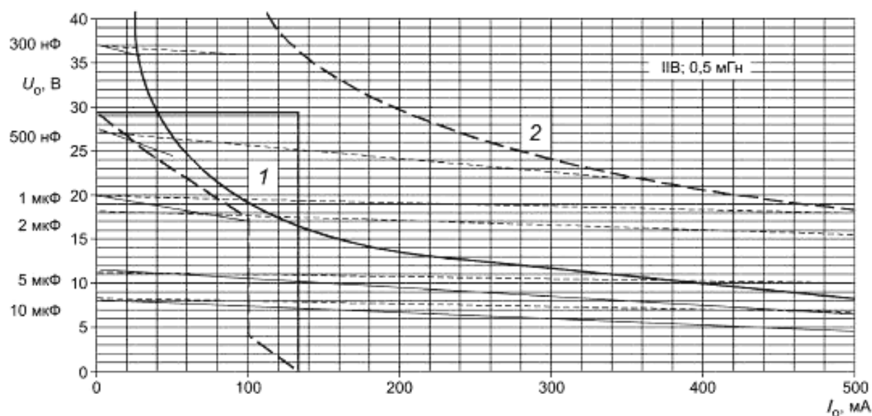
Рисунок С.6а — Сложение значений тока
