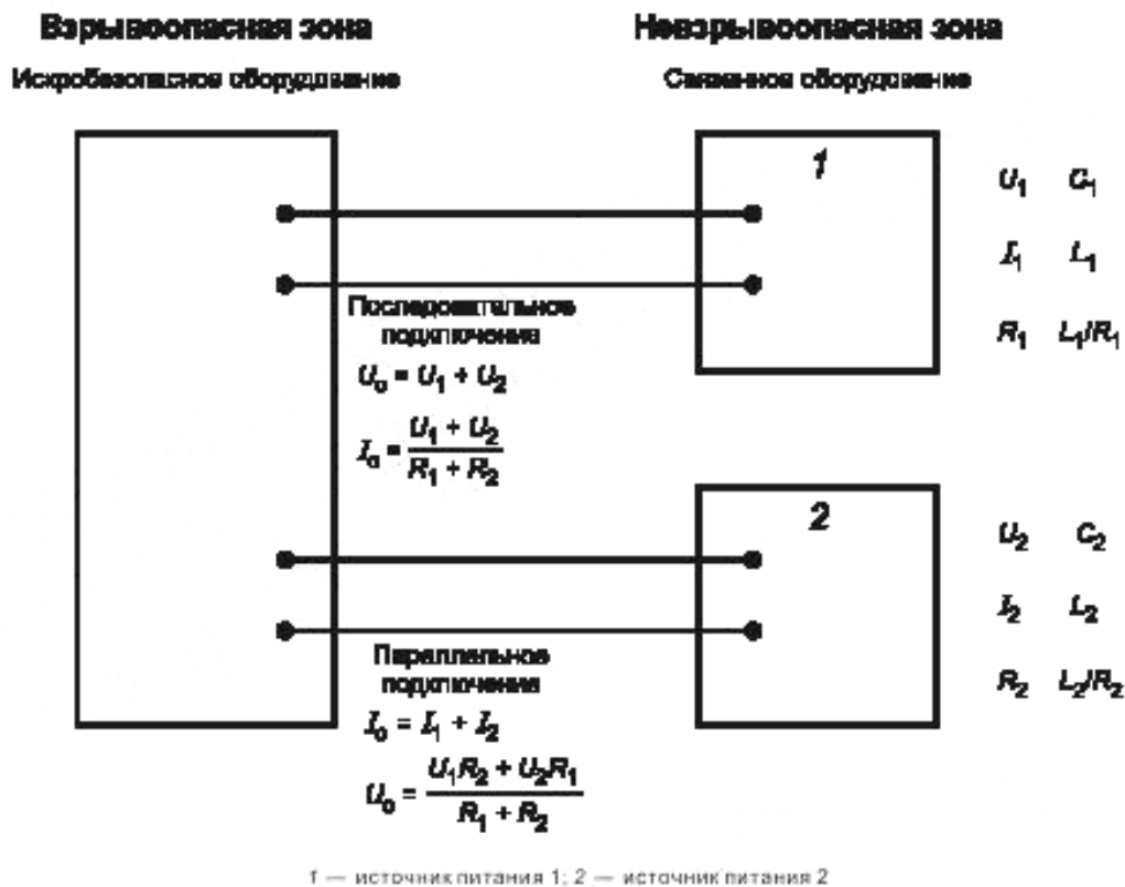
Рисунок В.3 — Произвольно подключенные источники питания
