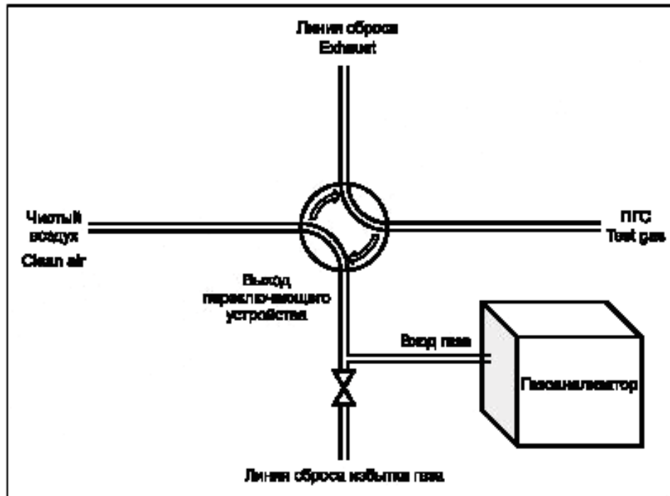
Рисунок В.1 — Схематическое изображение испытательной установки
