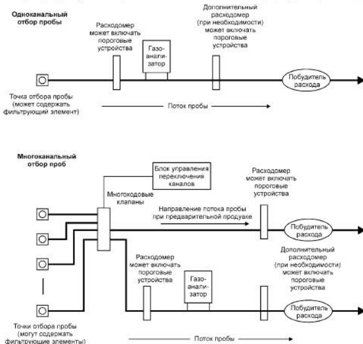
Рисунок А.2 — Типичные конфигурации пробоотборных линий
