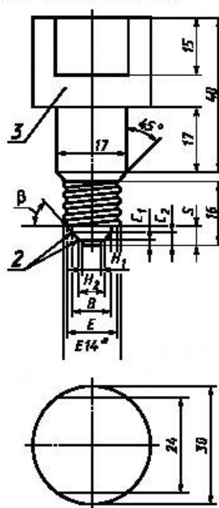
Испытательный цоколь В
