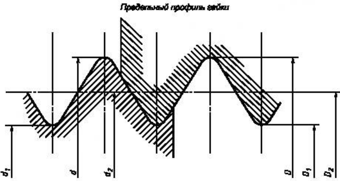
Предельный профиль винта
