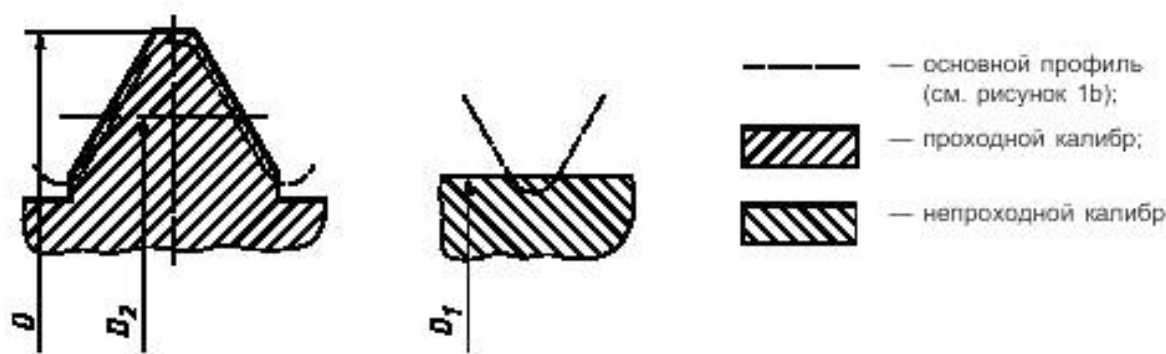
Калибры для гайки
