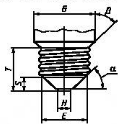
Испытательные цоколя E14 и E27
