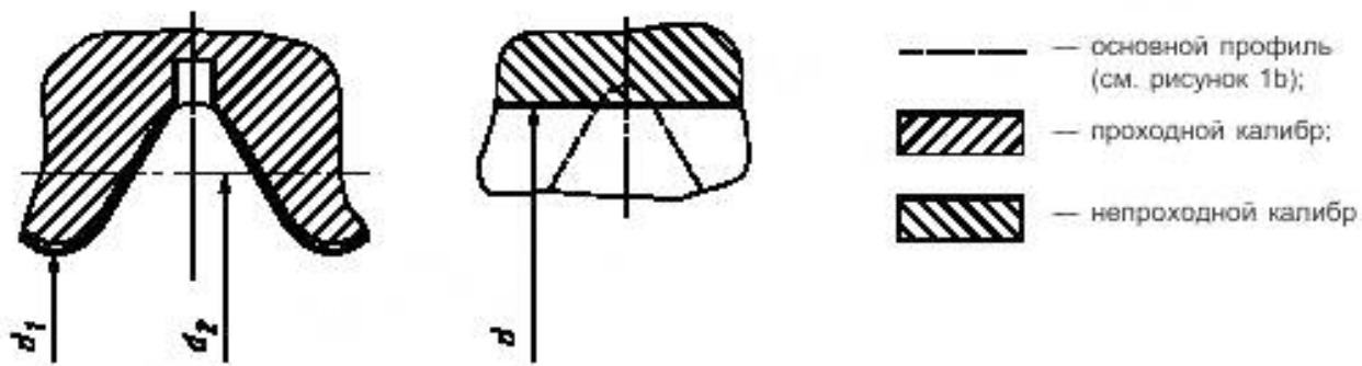
Калибры для винта
