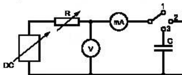
Рисунок 1 — Испытательная установка для выдержки при постоянном напряжении
