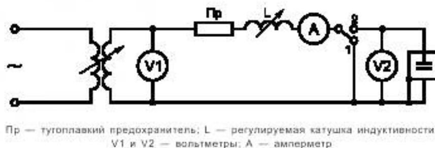
Рисунок 2 — Испытательная установка для разрушающего испытания переменным напряжением
