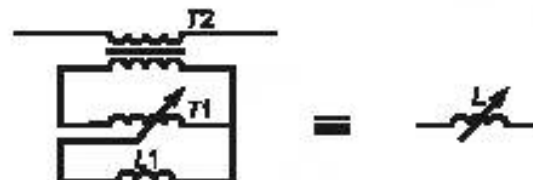
Рисунок 3 — Устройство для получения регулируемой индуктивности L , показанной на рисунке 2
