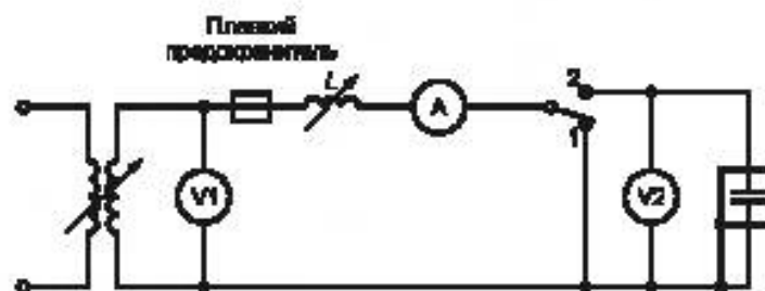
Рисунок 2 — Испытательная установка для разрушающего испытания переменным напряжением
