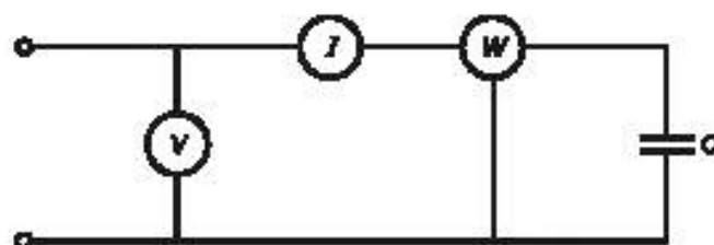
Рисунок 4 — Испытательная схема для измерения емкости и коэффициента мощности
