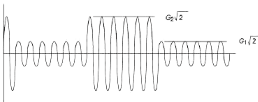
Рисунок 12 — Испытательная осциллограмма
