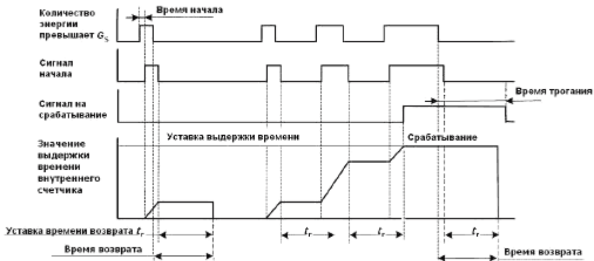
Рисунок 6 — Характеристика, поясняющая время возврата реле
