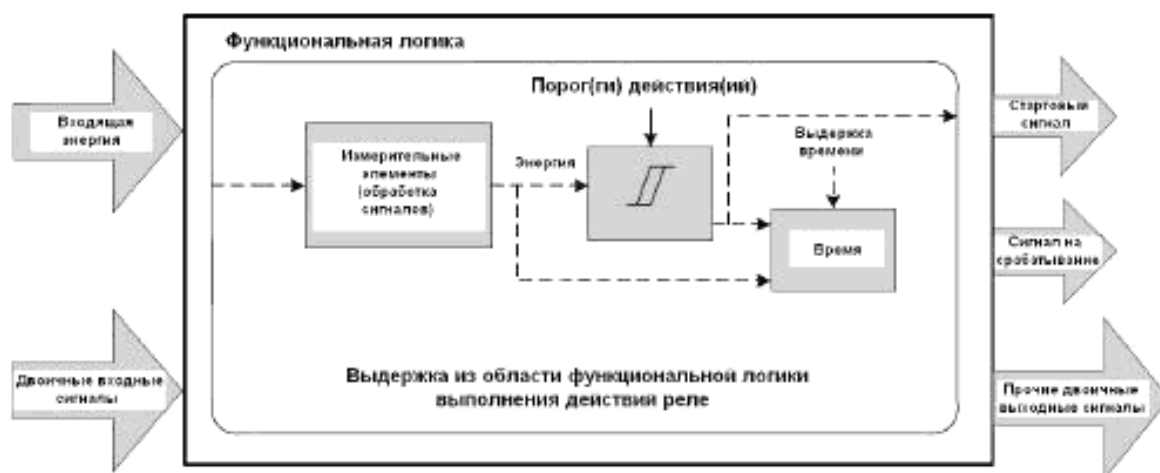
Рисунок 1 — Функциональный блок диаграмм выполнения защиты
