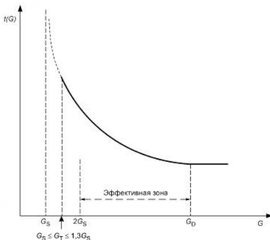
Рисунок 4 — Зависимая характеристика времени
