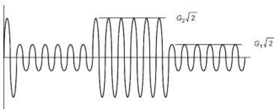
Рисунок 12 — Испытательная осциллограмма характеристической величины
