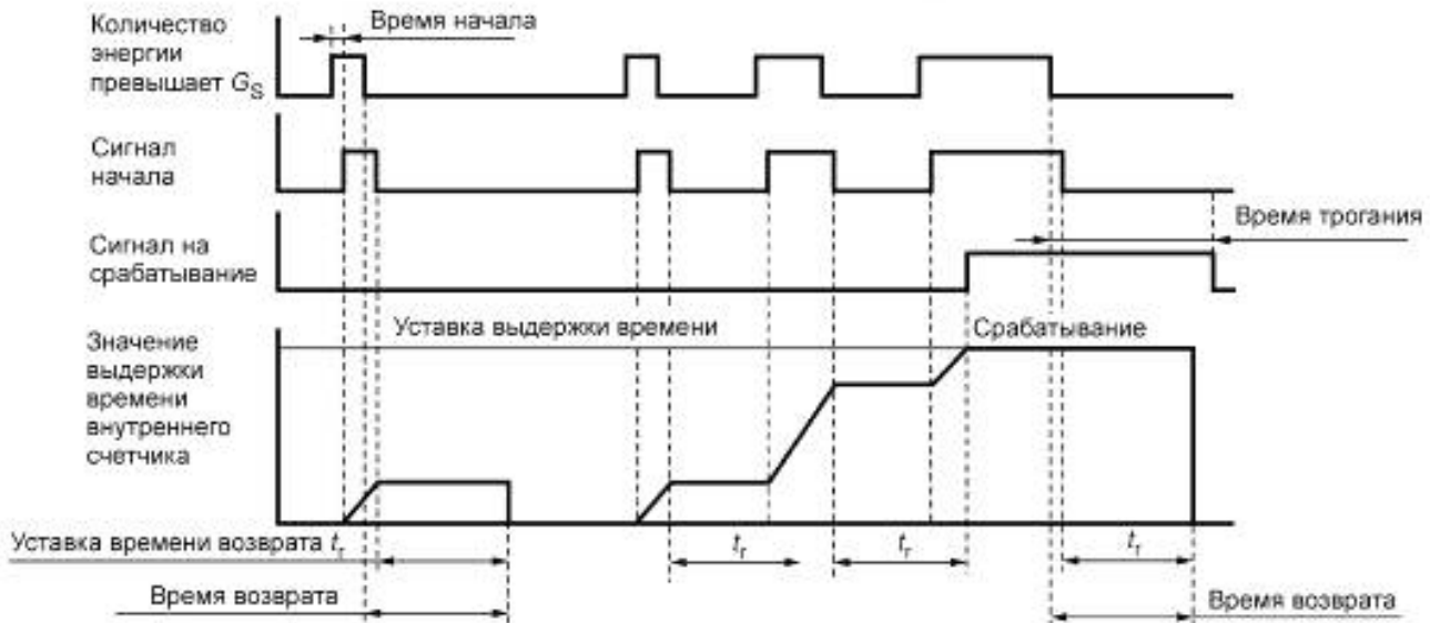
Рисунок 5 — Характеристика, поясняющая время возврата реле
