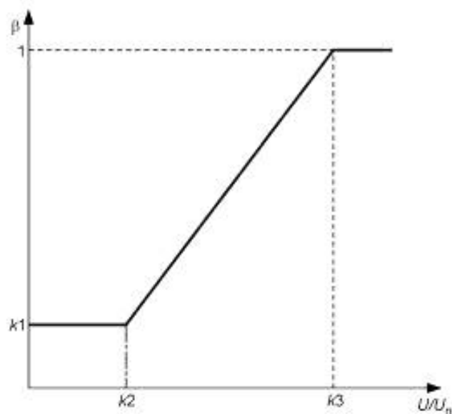
Рисунок 9 — Характеристика ограничения напряжения
