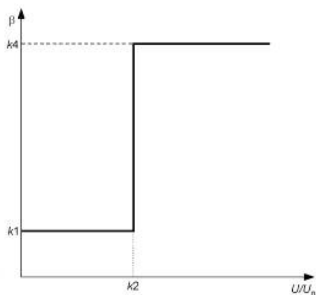
Рисунок 10 — Характеристика управляющего напряжения
