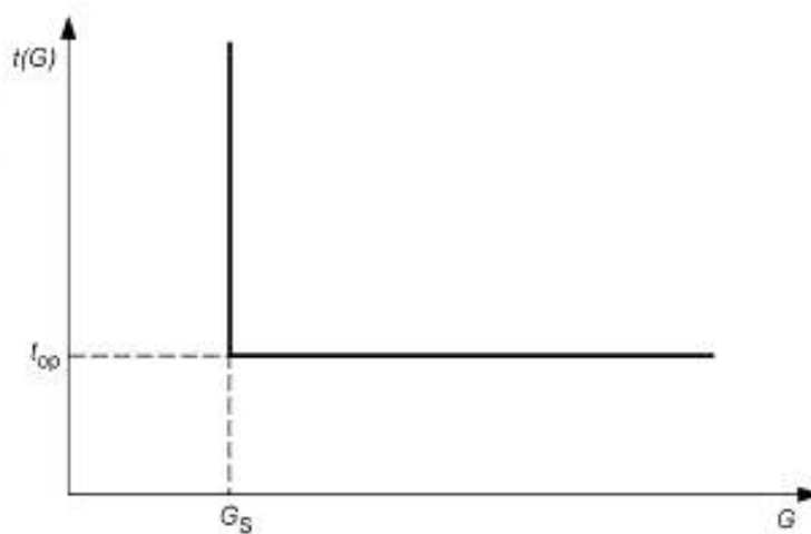
Рисунок 2 — Независимая характеристика времени реле сверхтока
