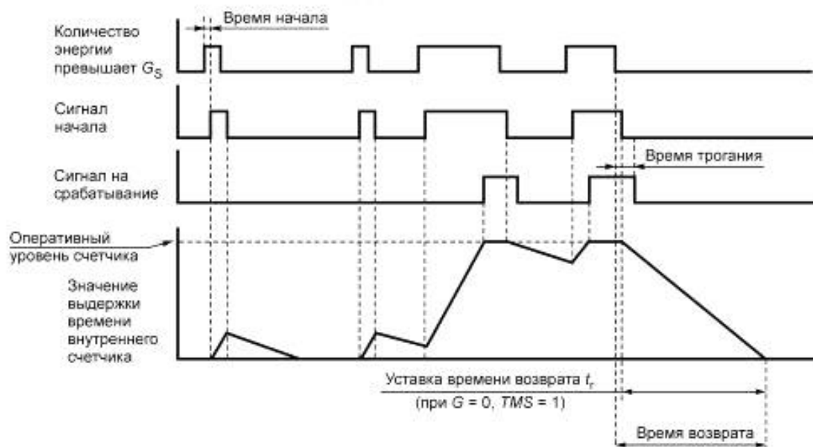
Рисунок 7 — Зависимая характеристика времени возврата
