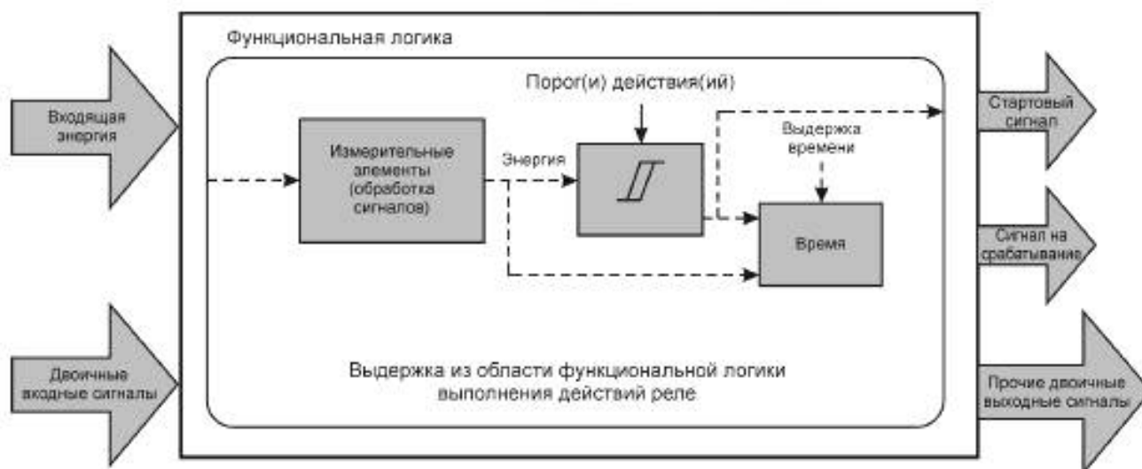
Рисунок 1 — Функциональный блок диаграмм выполнения защиты
