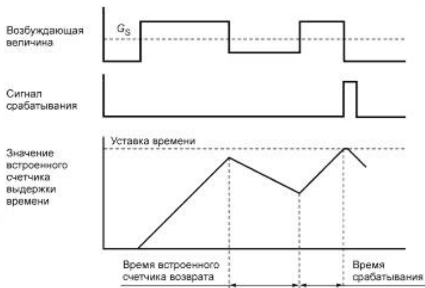
Рисунок В.1 — Определение зависимости времени возврата
