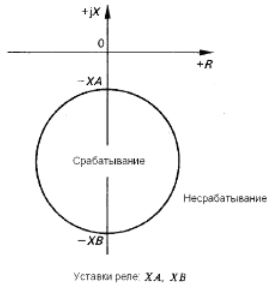
Рисунок 1f — Круговая смещенная характеристика
