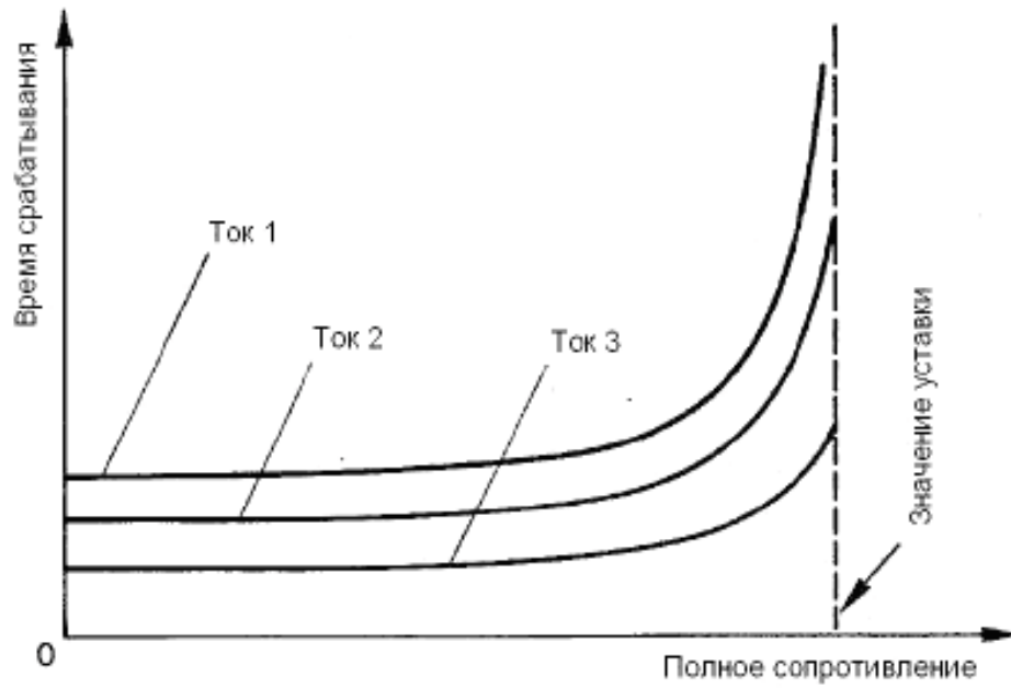
Рисунок 5 – Время срабатывания в нормальных условиях
