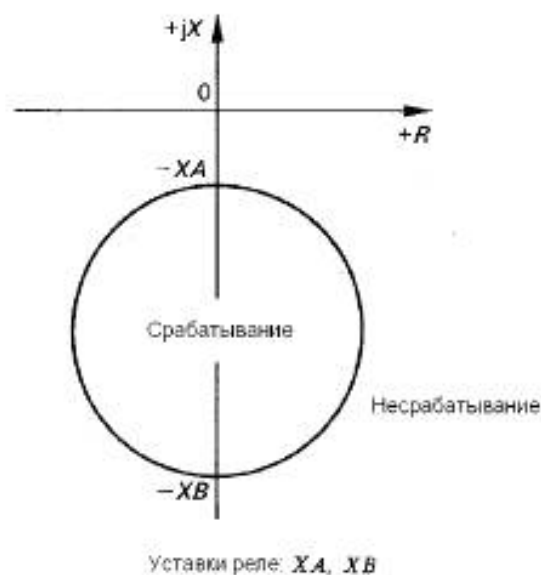
Рисунок 1f — Круговая смещенная характеристика
