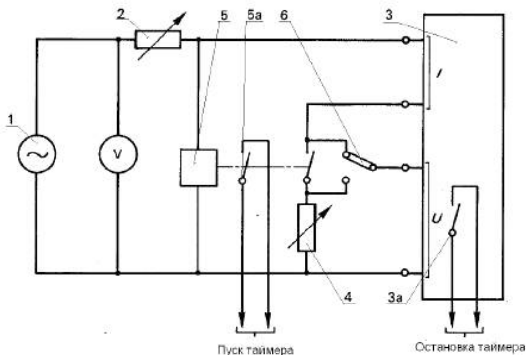
1 — стационарный источник напряжения; 2 — полное сопротивление регулируемого источника Z_s ; 3 — испытуемое реле; 3а — выходной контакт; 4 — регулируемое полное сопротивление Z_s , измеряемое посредством реле; 5 — управляющее устройство точечного переключения; 5а — выключатель мгновенной подачи входных воздействующих величин; 6 — переключающий элемент
