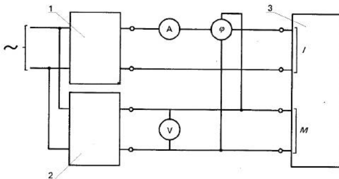
1 — регулируемый источник тока; 2 — регулируемый источник напряжения со сдвигом фаз от 0 до 360°; 3 — испытуемое реле
