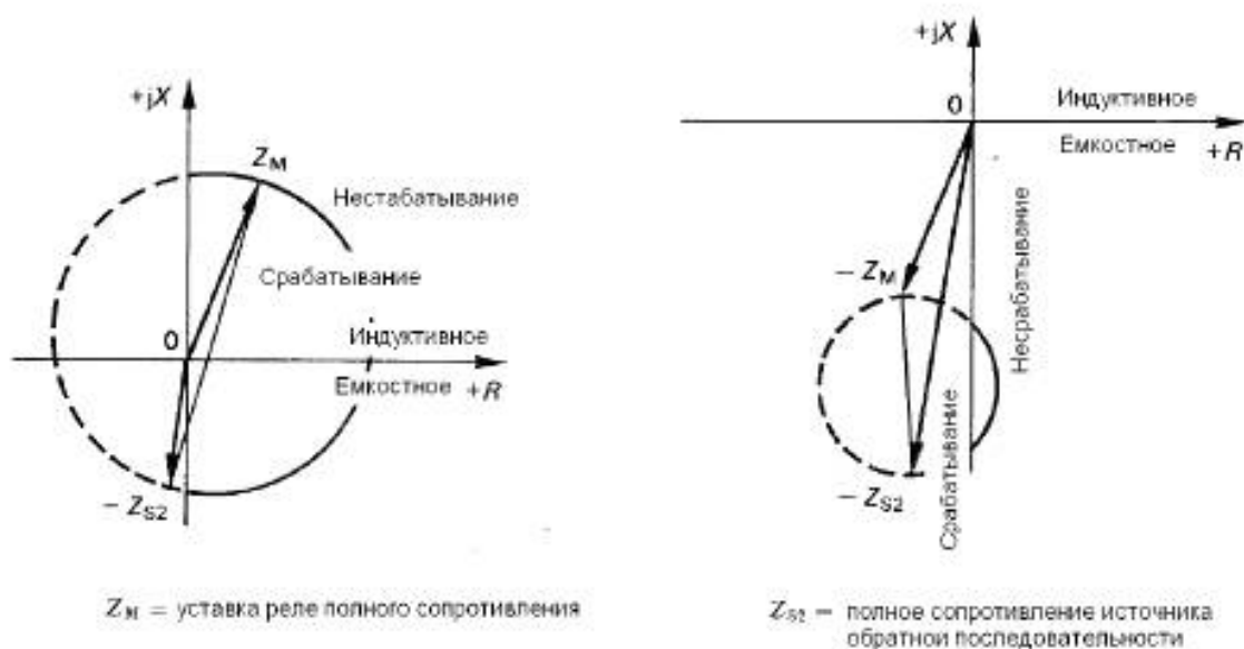
Рисунок 1е — Круговая характеристика межфазного повреждения прямого направления (влево) и обратного направления (вправо)
