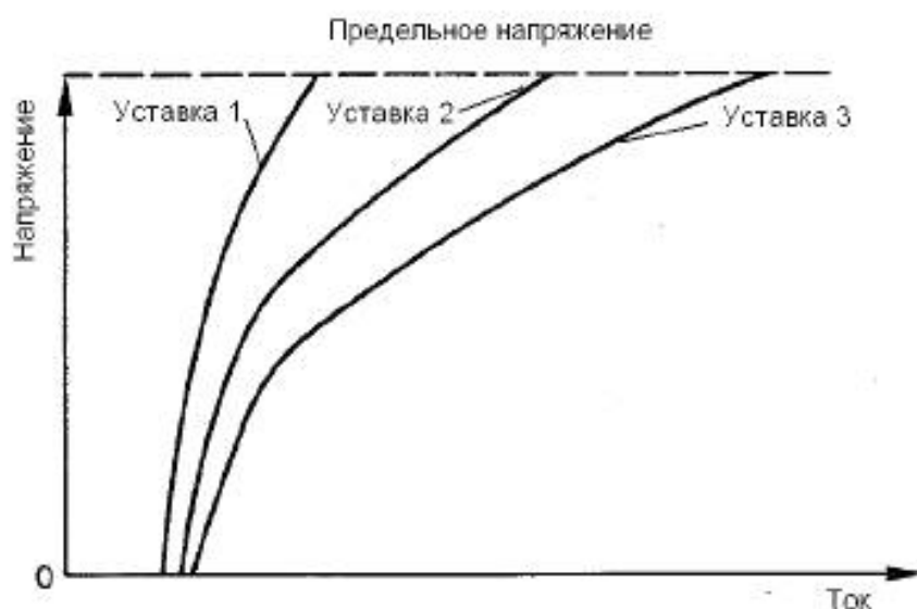
Рисунок 3 — Характеристика срабатывания U = f(I)
