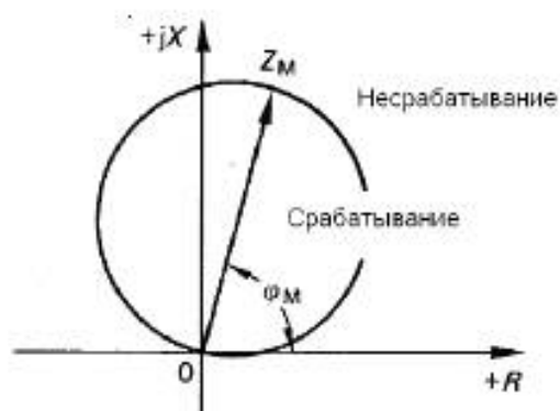
Рисунок 1а — Круговая характеристика
