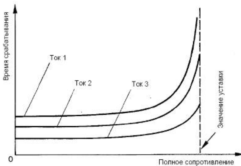
Рисунок 5 — Время срабатывания в нормальных условиях
