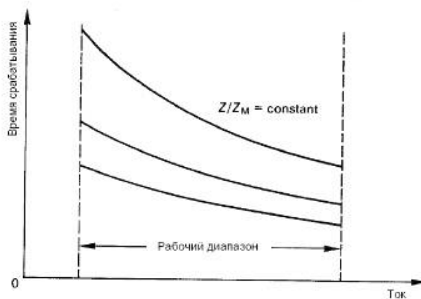
Рисунок 5 — Время срабатывания в нормальных условиях
