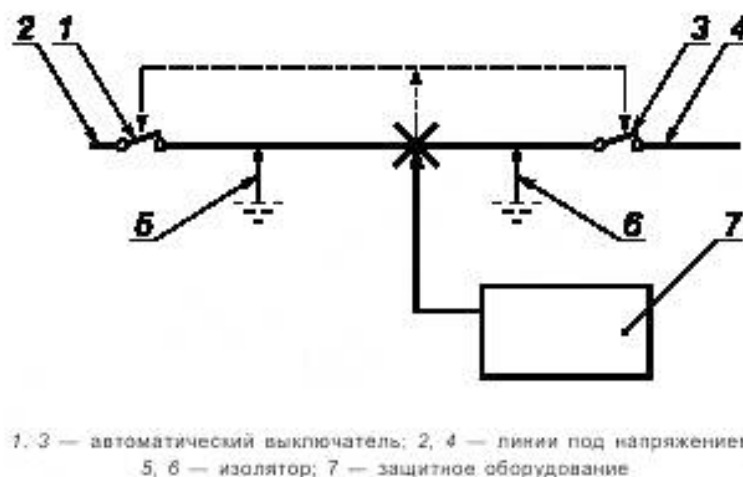
Рисунок L.2 — Линии, находящиеся под напряжением, механически изолированы изоляторами или электромеханически автоматическим выключателем; отключенные линии в последующем обезопасены заземлением
