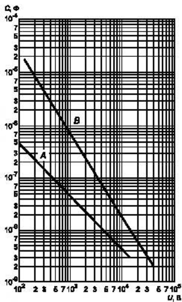
Рисунок 1.2 — Уровень зарядки конденсатора в условиях нормальной эксплуатации и в условиях первичного повреждения
