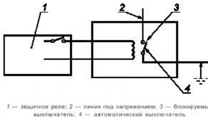
Рисунок L.1 — Упрощенная схема блокировки, на которой представлено защитное реле, управляющее автоматическим выключателем на его размыкание; отключенная линия в последующем обезопасена заземлением
