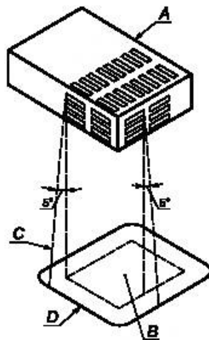
Рисунок 3 — Размещение и размеры негорючего огнезащитного ограждения
