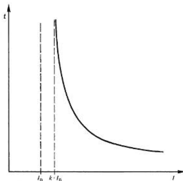
Пример характеристической кривой реле в «холодном» состоянии
