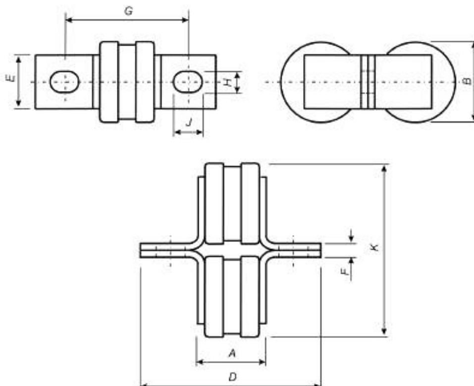
Рисунок СС.1 — Одинарный корпус плавкой вставки
