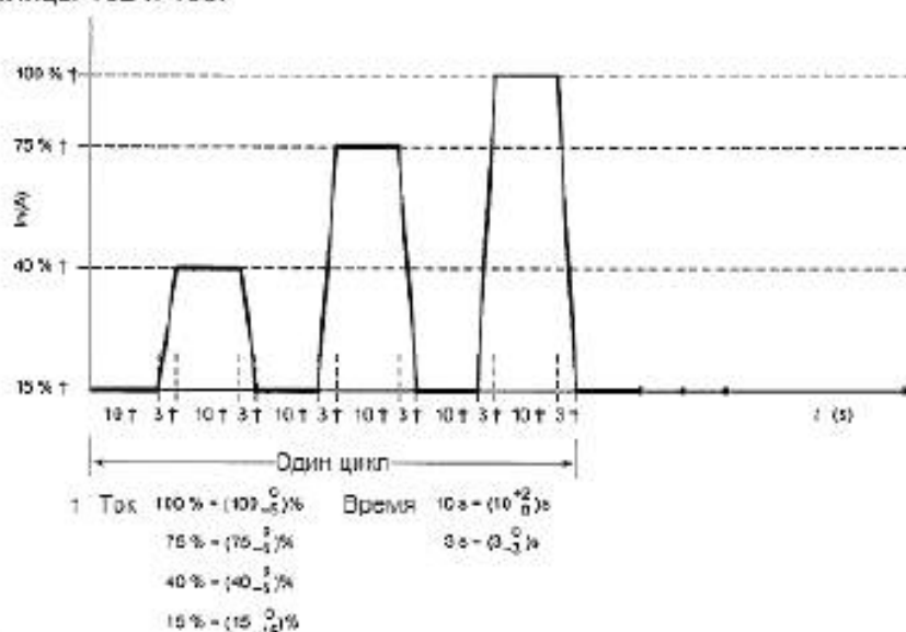
Рисунок 101 — Ток испытательного цикла
