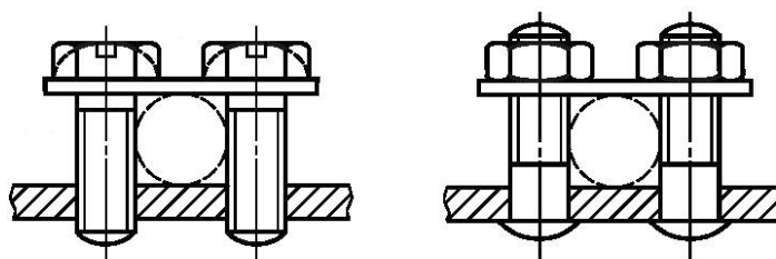
Рисунок 14е — Пластиначные выводы
