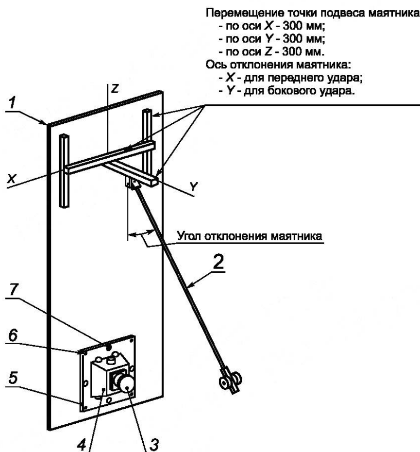
1 — панель из фанеры; 2 — маятник; 3 — образец; 4 — монтажная плата; 5 — нижняя плата; 6 — фиксирующие штыри; 7 — винты крепления
