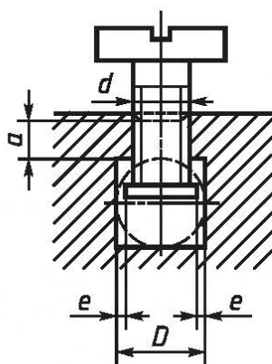
Зажим с прижимной пружиной
