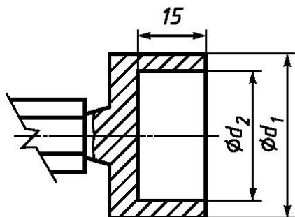
Калибр А для проверки диаметра d_1
