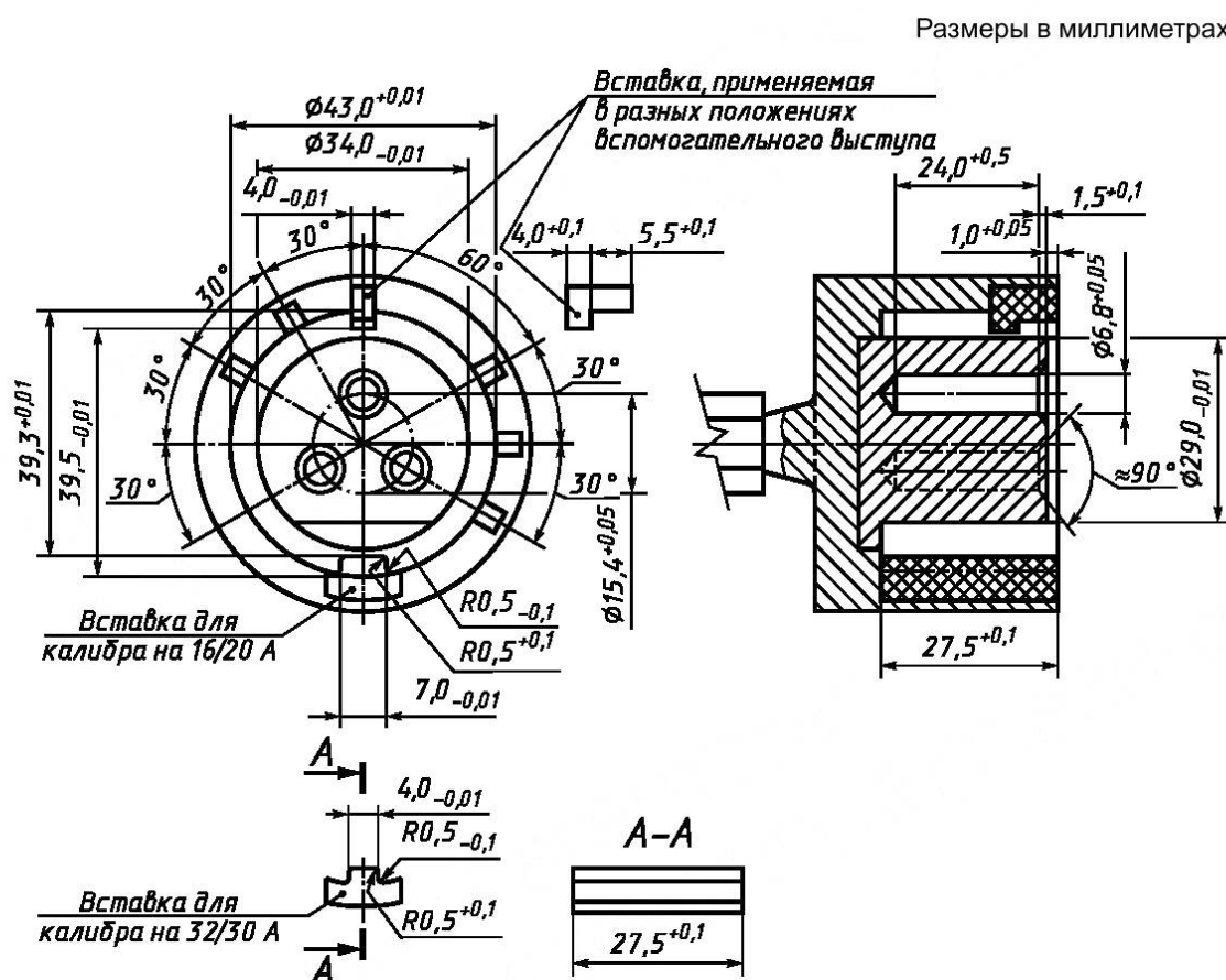
Рисунок 111 — Штепсельные или переносные розетки на токи 16/20 и 32/30 А и номинальное рабочее напряжение не более 50 В. Калибры для проверки прочности оболочки из термопластичного материала в теплых и влажных условиях
