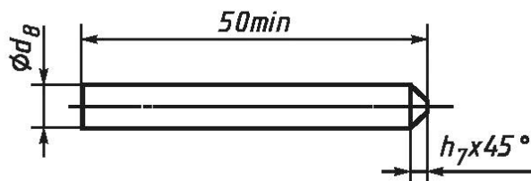
Рисунок 105 — Калибр для проверки фазных гнезд
