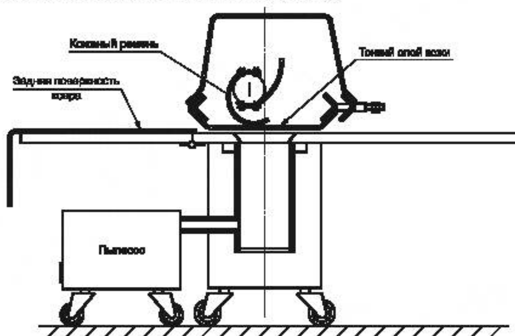
Рисунок 19 — Машина для выбивания ковра
