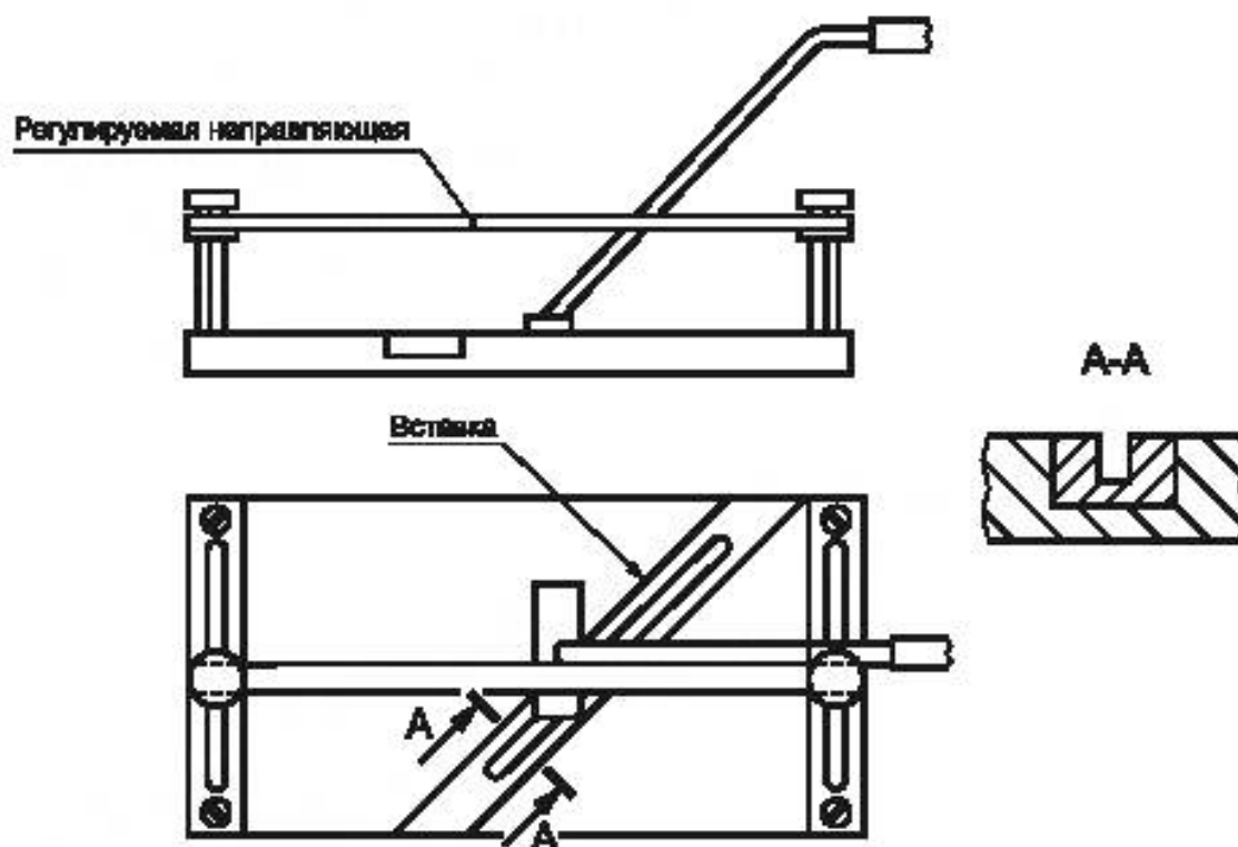
Рисунок 18 — Испытательная пластина со щелью
