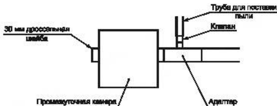
Рисунок 10 — Подсоединение трубки к отверстию
