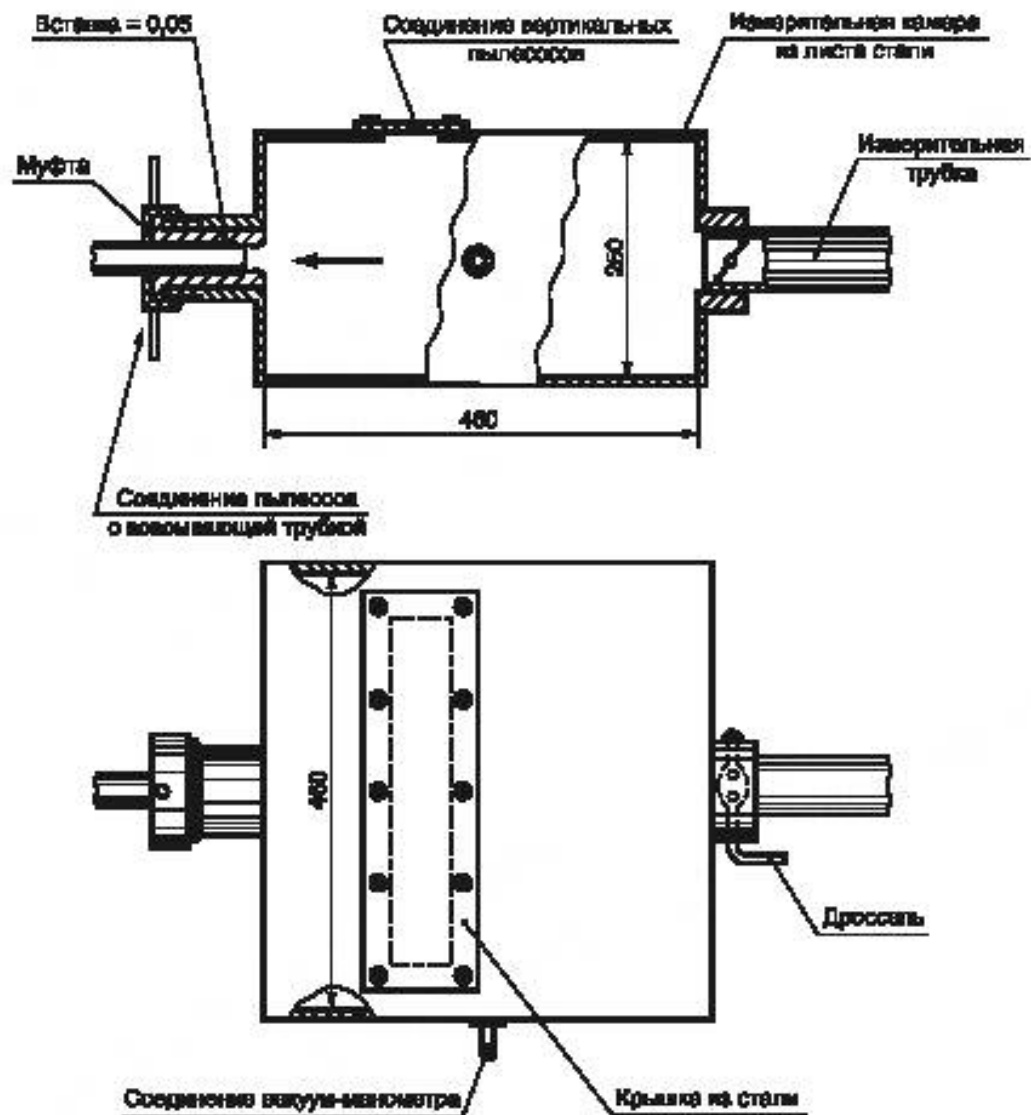
Рисунок 23 — Измерительная камера для альтернативного оборудования А
