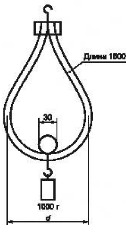
Рисунок 16 — Подготовка шлангов для испытания на гибкость
