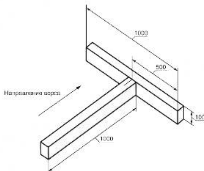
Рисунок 1 — Т-образная конструкция
