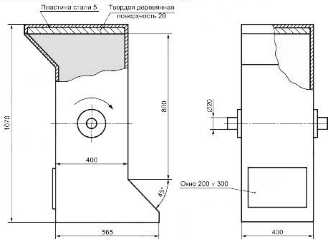
Рисунок 28 — Барабан для испытания на воздействие
