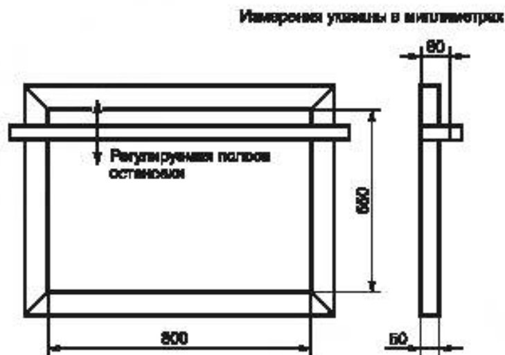
Рисунок 5 — Рама для испытательной подушки
