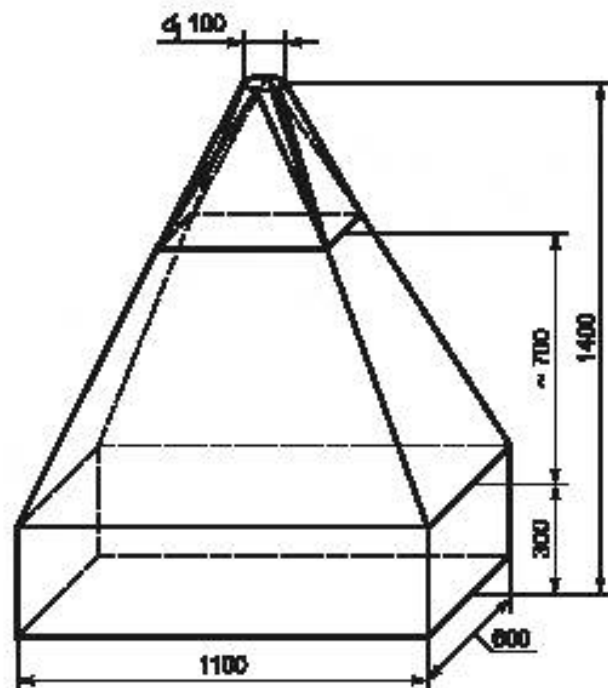
Рисунок 25 — Испытательный кожух
