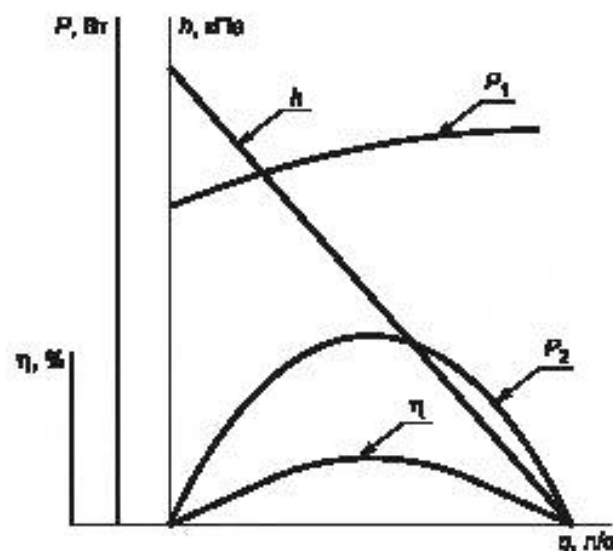
Рисунок 9 — Кривые показателей воздуха
