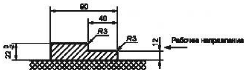
Рисунок 14 — Профиль порога
