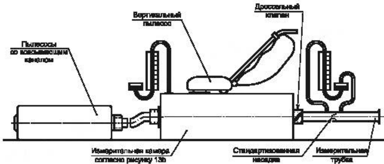
Рисунок 22 — Альтернативное оборудование А для испытания параметров воздуха
