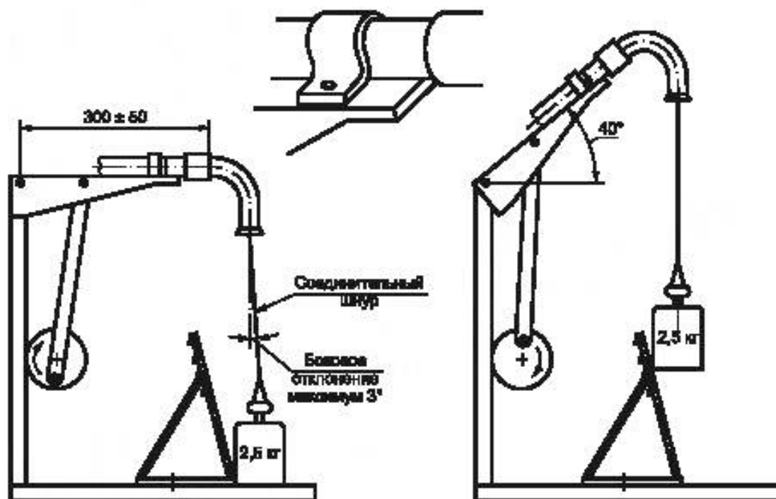
Рисунок 17 — Оборудование для повторного изгиба шланга
