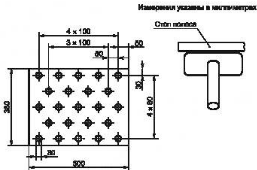
Рисунок 6 — Трафарет для распределения волокон на обивке
