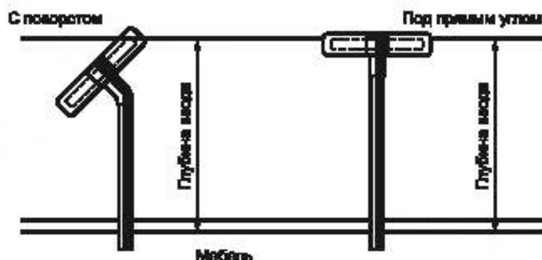
Рисунок 12 — Глубина ввода
