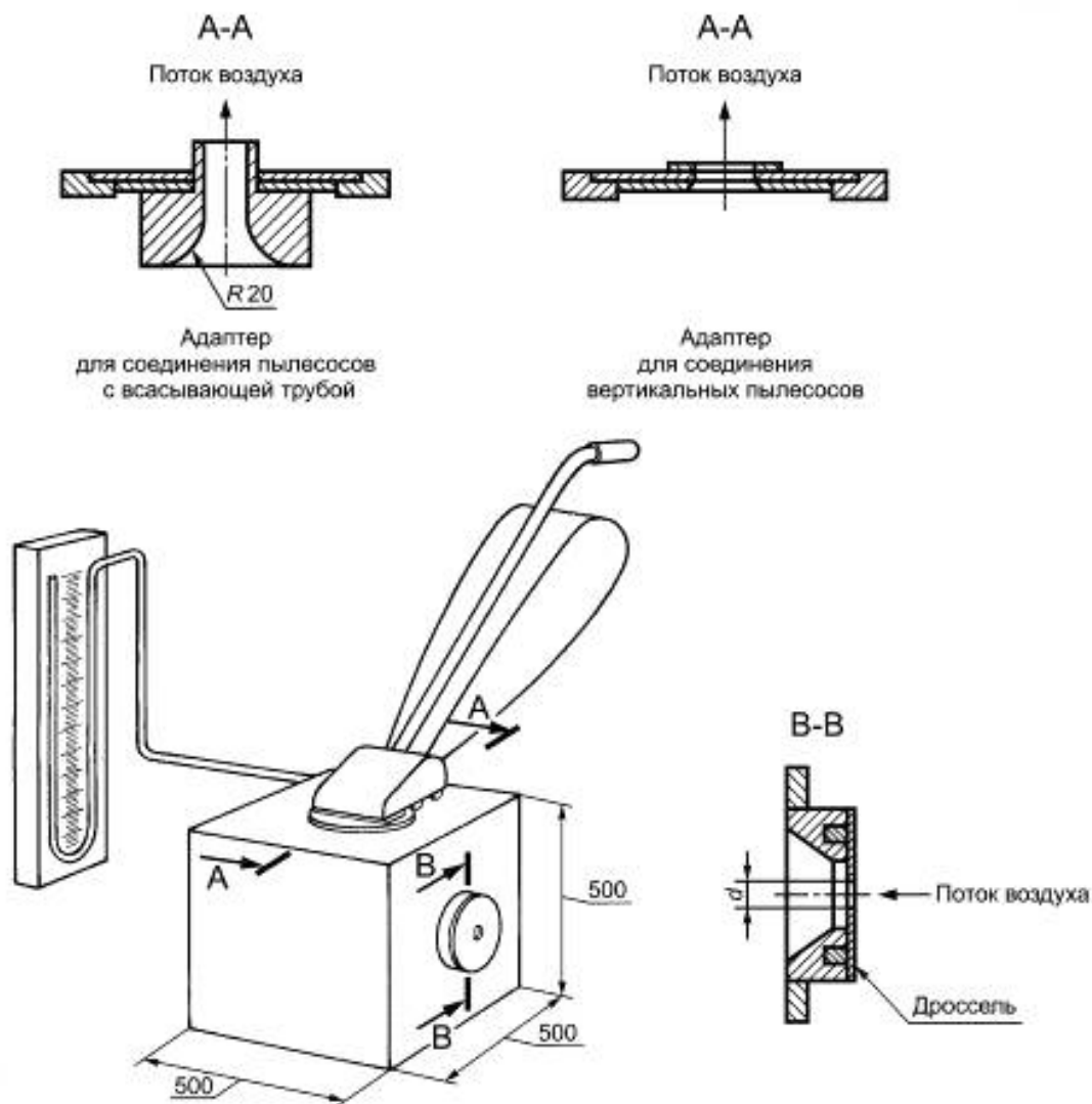
Рисунок 24 — Альтернативное оборудование В для испытания параметров воздуха
