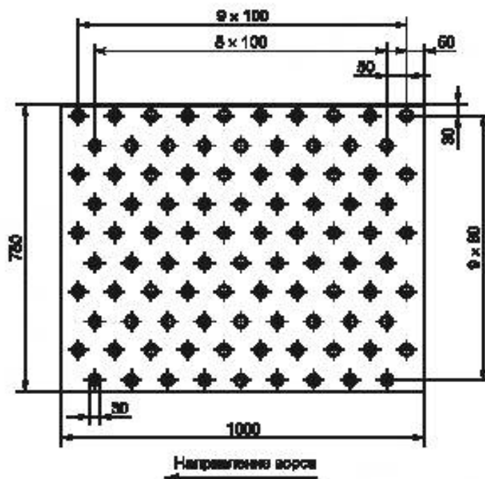
Рисунок 3 — Трафарет для распределения волокон по испытательным коврам
