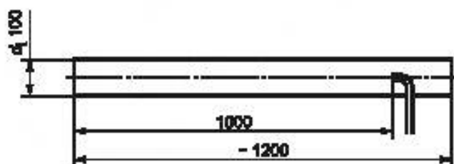
Рисунок 27 — Выхлопной канал с выборкой для исследования
