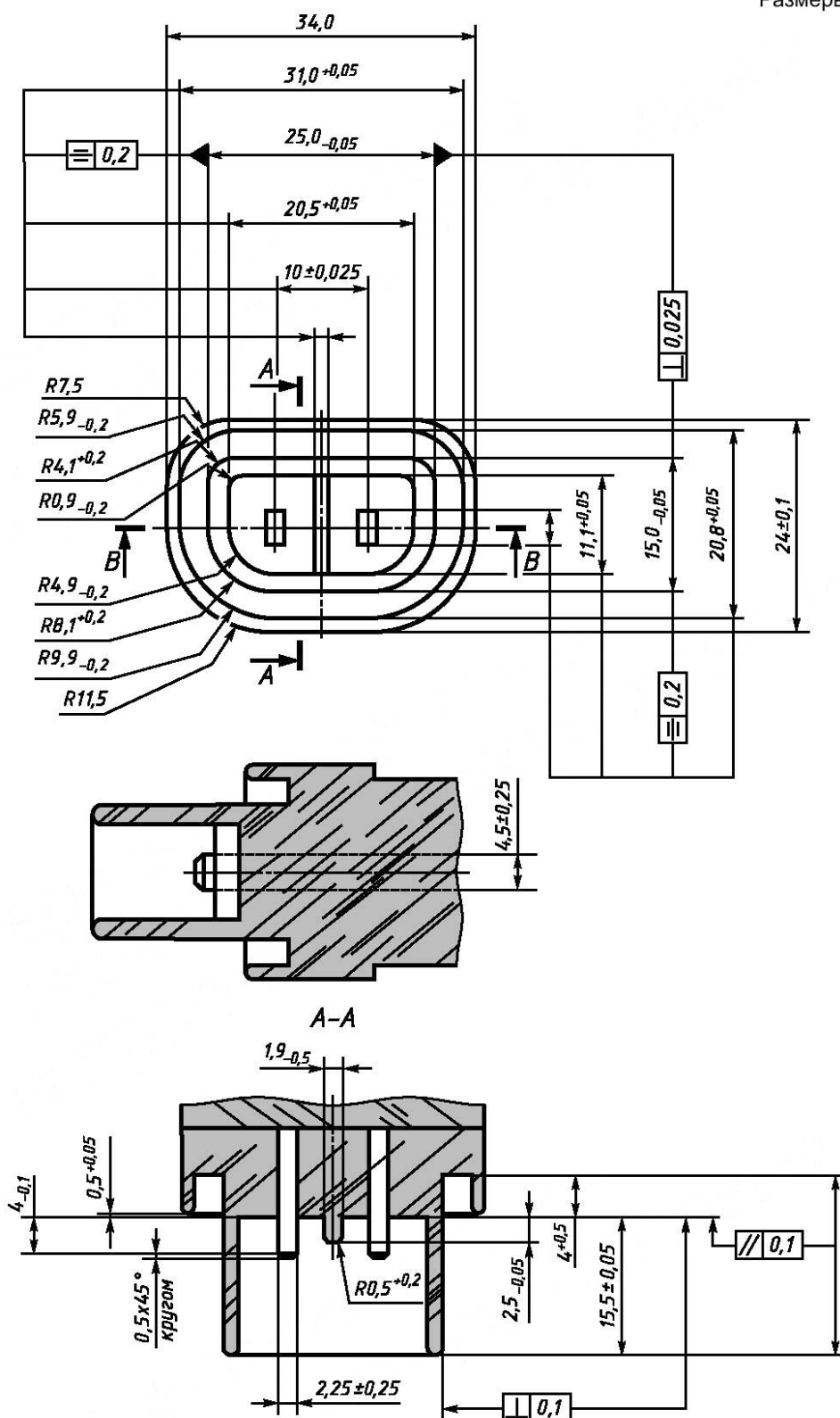
Рисунок 1А — «Проходной» калибр для соединителей согласно стандартному листу С (см. 9.1)
