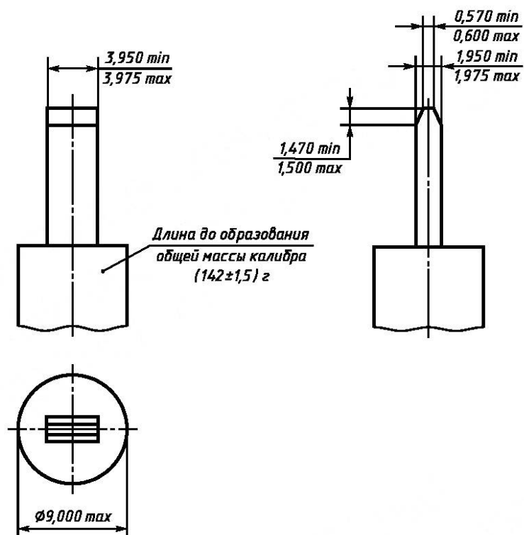
Рисунок 4 — Вытягивающий калибр (см. 13.5)
