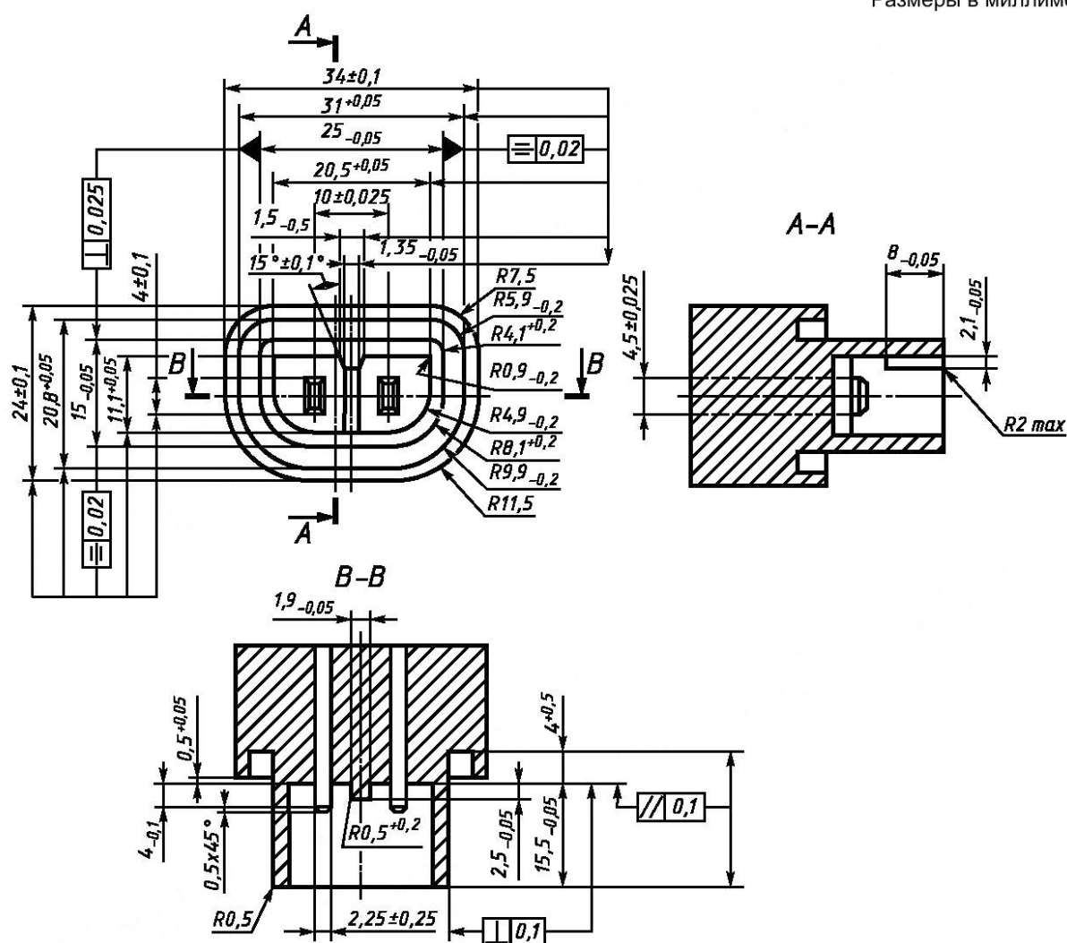
Рисунок 1 — «Прходной» калибр для соединителей согласно стандартному листу А (см. 9.1)
