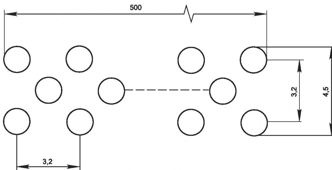
Рисунок 2 — Фронтальная поверхность рабочей части горелки
