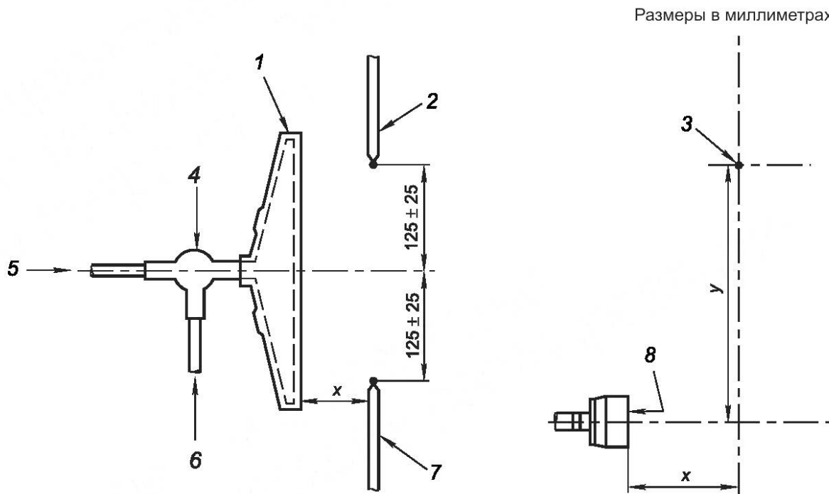
1 — горелка; 2 — термопара А; 3 — кончик термопары; 4 — смеситель Вентури; 5 — подача воздуха; 6 — подача пропана; 7 — термопара В; 8 — фронтальная поверхность рабочей части горелки
