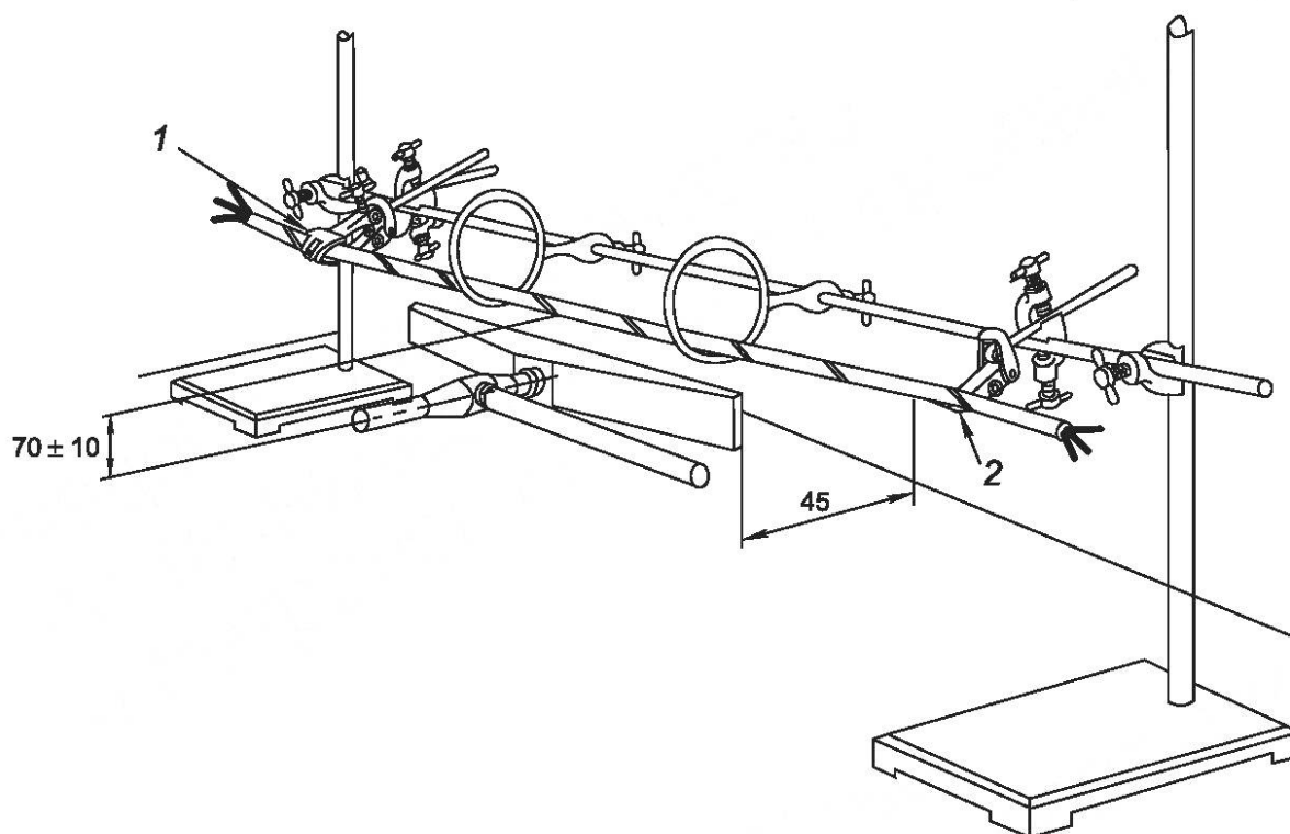
Рисунок 1 — Пример поддерживающего устройства
