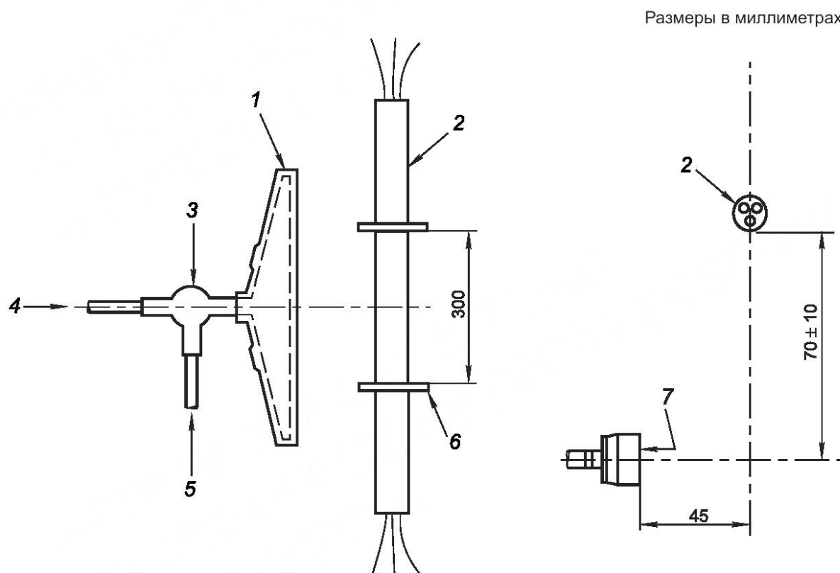
1 — горелка; 2 — образец кабеля; 3 — смеситель Вентури; 4 — подача воздуха; 5 — подача пропана; 6 — поддерживающие кольца; 7 — фронтальная поверхность рабочей части горелки
