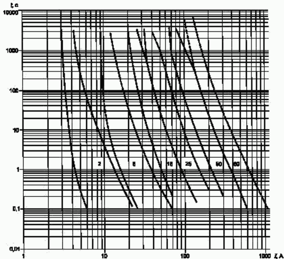
Рисунок А.1 — Время-токовые зоны для плавкого предохранителя
