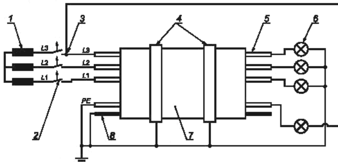
1 — трансформатор; 2 — плавкий предохранитель (2 А); 3 — подсоединение к линии L3 (или L1, или L2); 4 — поддерживающие кольца; 5 — испытываемая жила или группа жил; 6 — нагрузочный индикаторный прибор (например, лампа); 7 — образец; 8 — металлический экран (если имеется); L1, L2, L3 — линии испытываемых жил или групп жил (L2, L3, если имеются); PE — жила заземления (если имеется)
