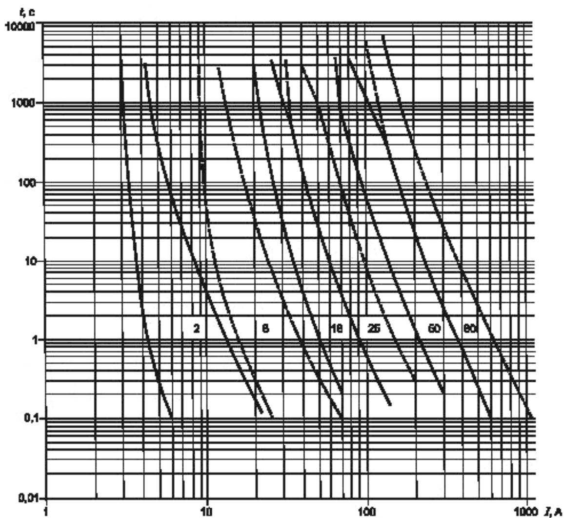
Рисунок А.1 — Время-токовые зоны для плавкого предохранителя
