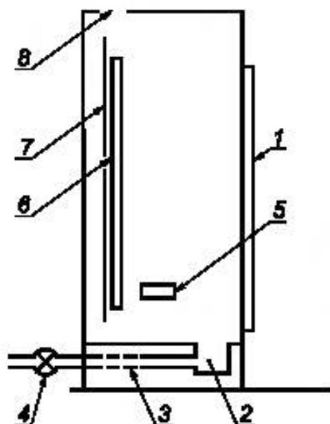
Рисунок 1а — Испытательная камера
