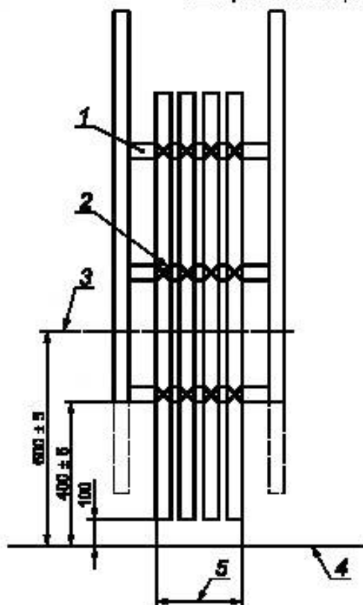
Рисунок 3 — Расположение горелки и стандартное размещение образца на лестнице
