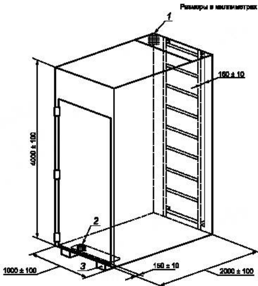
Рисунок 1а — Испытательная камера
