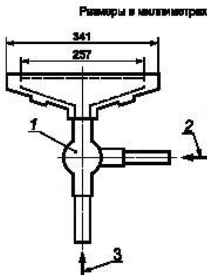
Рисунок 5а — Одиночная горелка, используемая при стандартной лестнице
