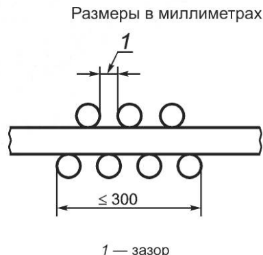
Рисунок 1 — Кабели, закрепленные на обеих сторонах лестницы с зазором (категория A F/R)
