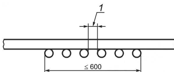
Рисунок 2 — Кабели, закрепленные на передней стороне широкой лестницы с зазором
