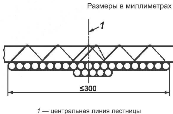
Рисунок 1 — Кабели, закрепленные на передней стороне лестницы без зазора (комплекты отрезков кабелей находятся в контакте)
