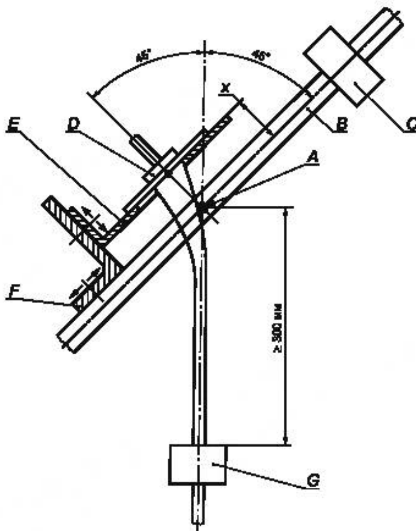
А – ось качания; В – качающийся элемент (рама); С – противовес; D – образец; E – регулируемая несущая плита; F – регулируемый кронштейн; G – груз
