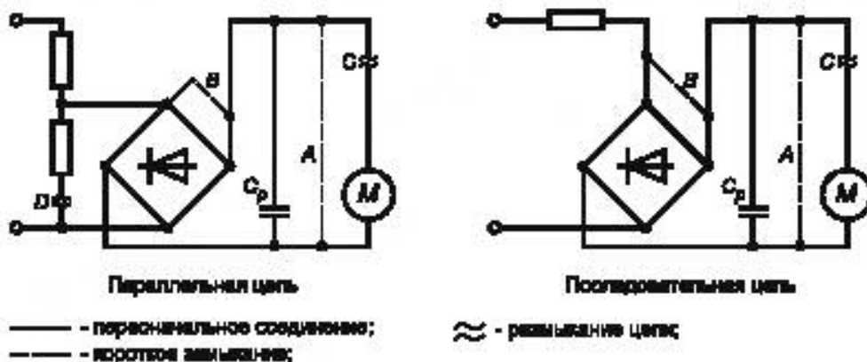
Рисунок I.1 – Имитация условий неисправности
