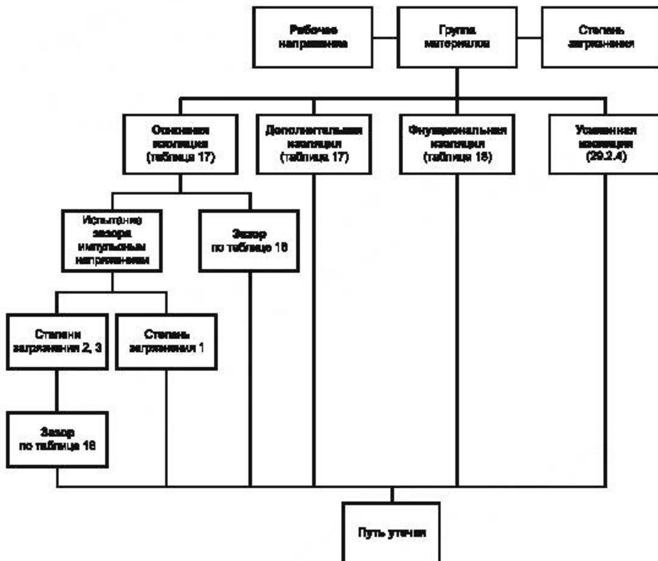
Рисунок L.2 – Последовательность для определения путей утечки
