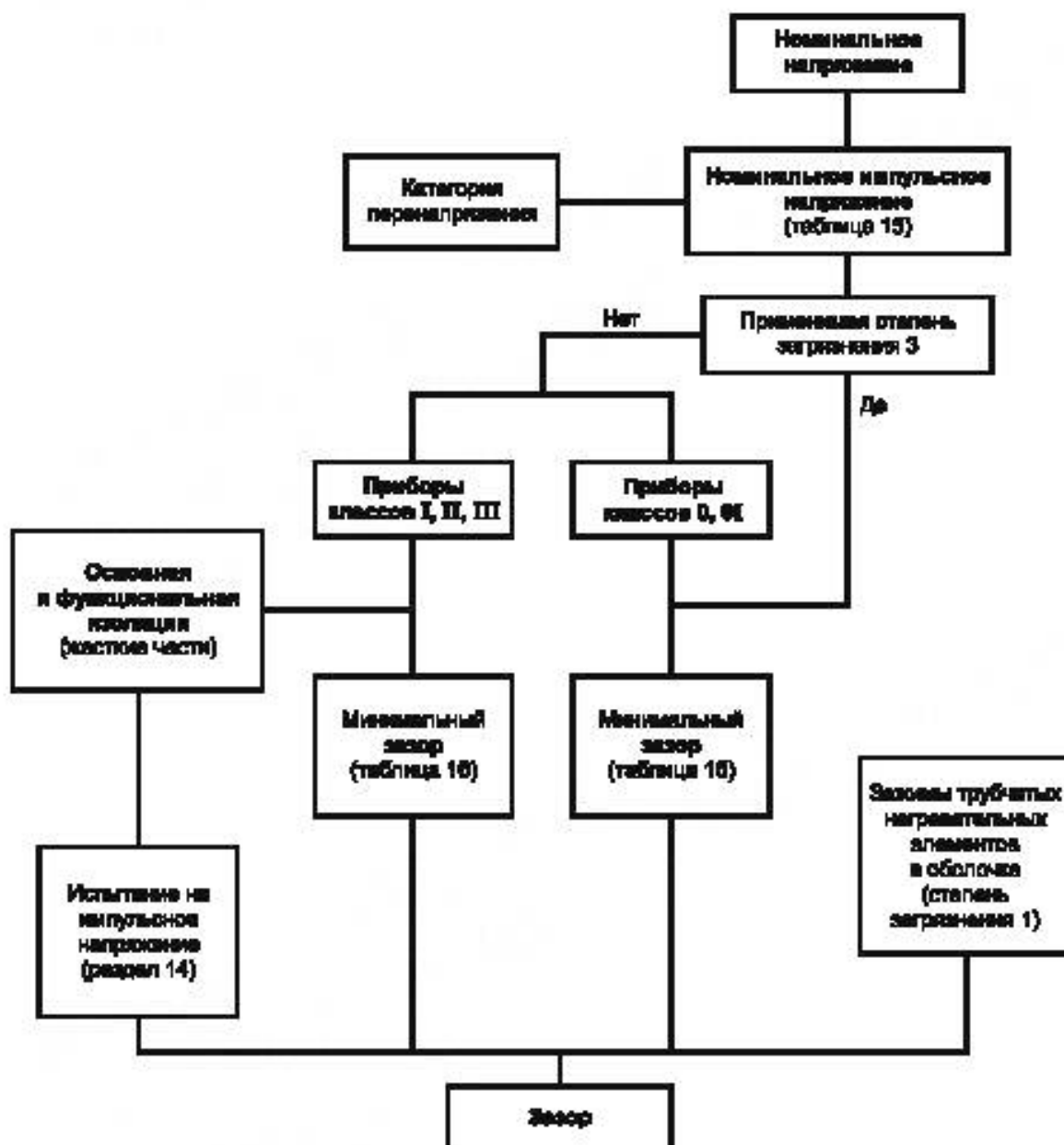
Рисунок L.1 – Последовательность для определения зазоров
