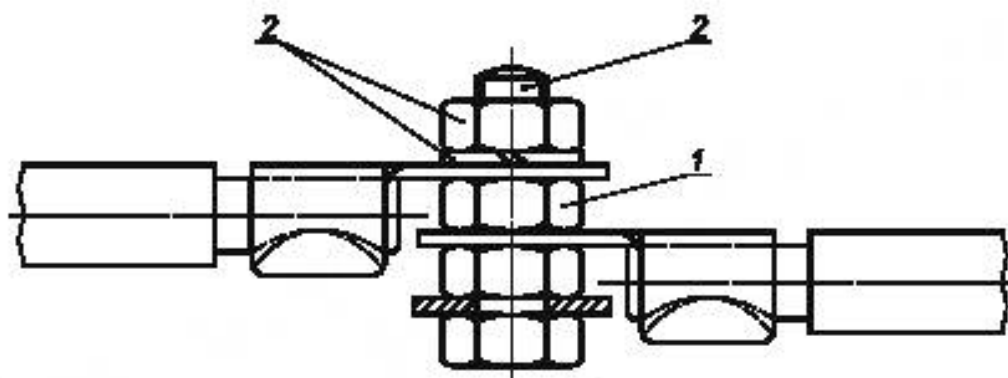
Рисунок 10 – Пример частей заземляющего зажима
