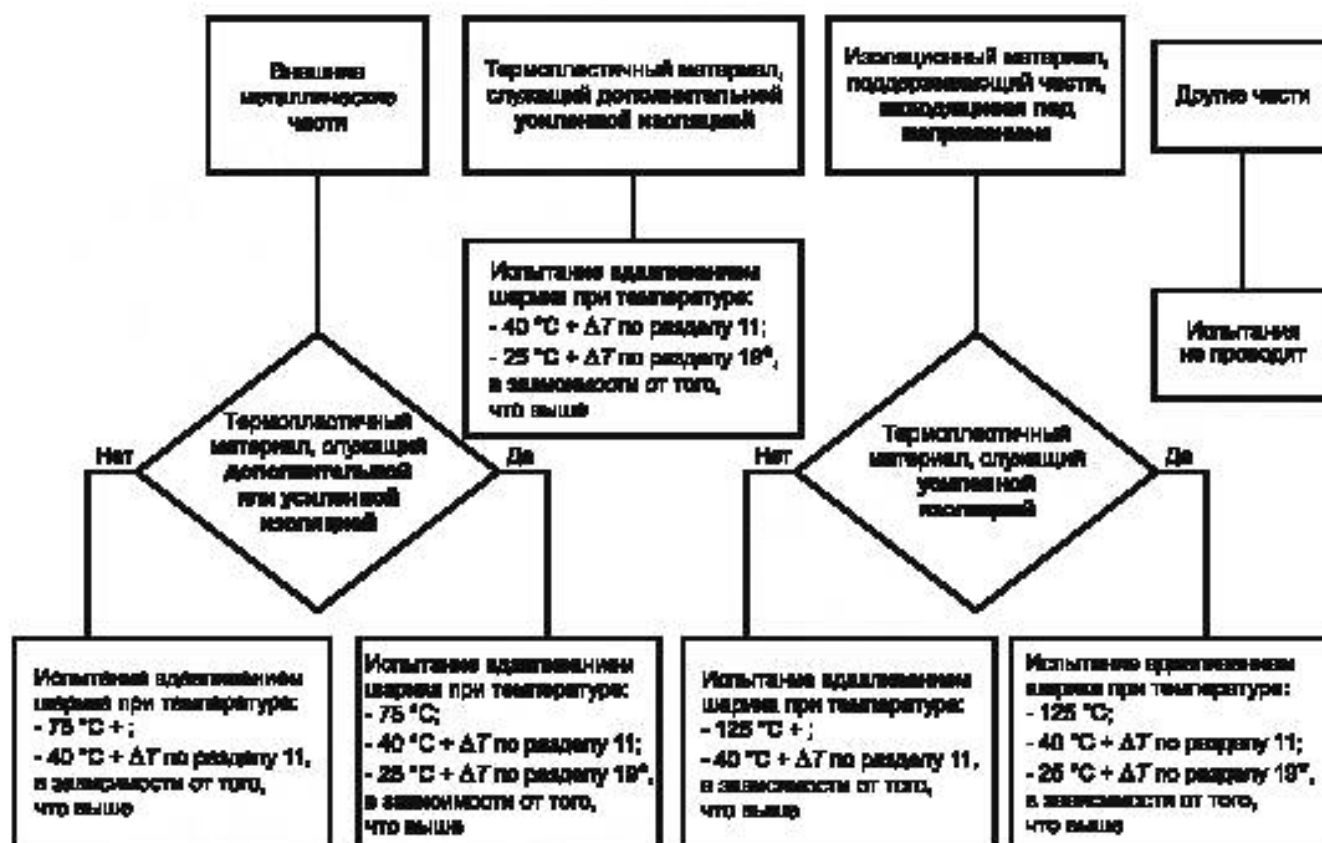
Рисунок О.1 – Испытания на теплостойкость
