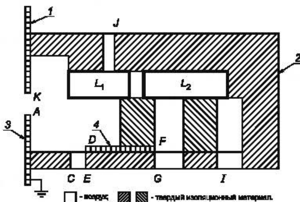
Рисунок 10 – Пример частей заземляющего зажима
