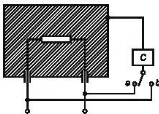
Рисунок 2 – Схема измерения тока утечки при рабочей температуре для однофазных приборов, кроме приборов класса II
