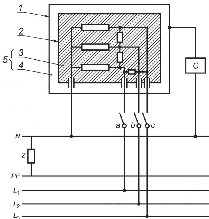
Рисунок 2 — Схема измерения тока утечки при рабочей температуре для однофазных приборов, кроме приборов класса II и частей конструкции класса II
