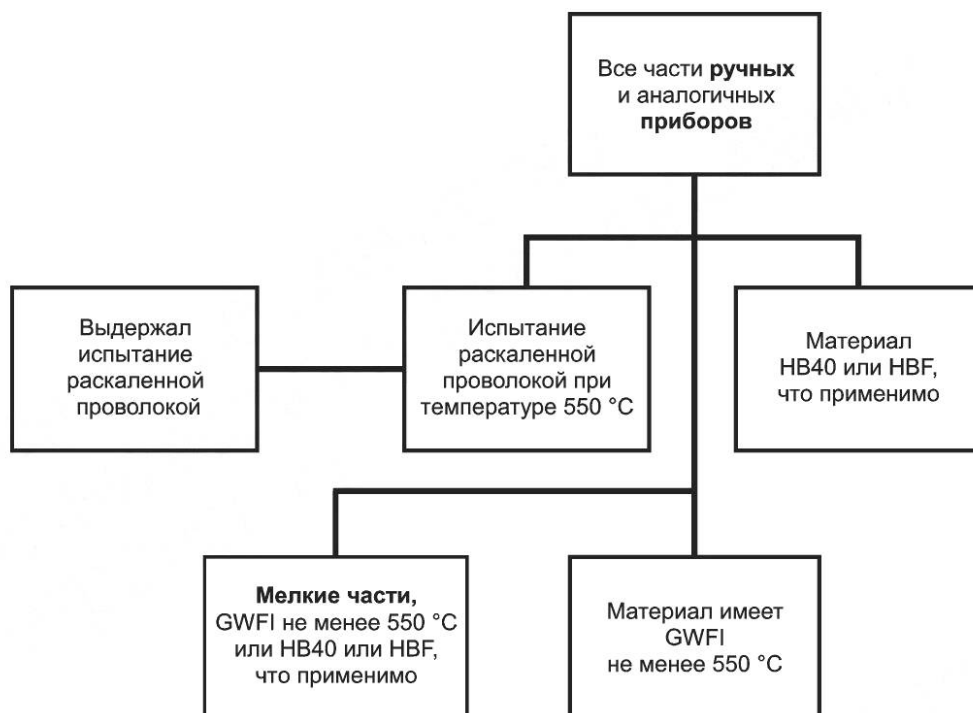
Рисунок O.2 — Выбор и последовательность испытаний на огнестойкость ручных приборов
