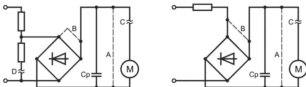
а) Параллельная цепь
