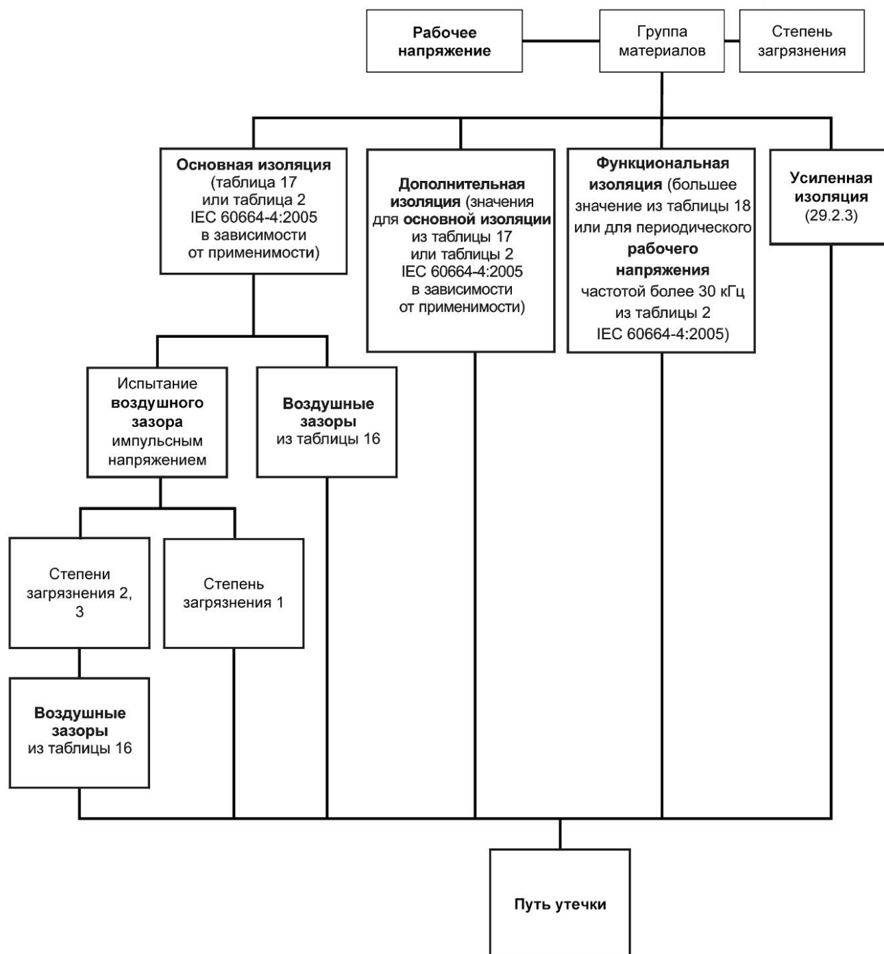
Рисунок L.2 — Алгоритм определения путей утечки
