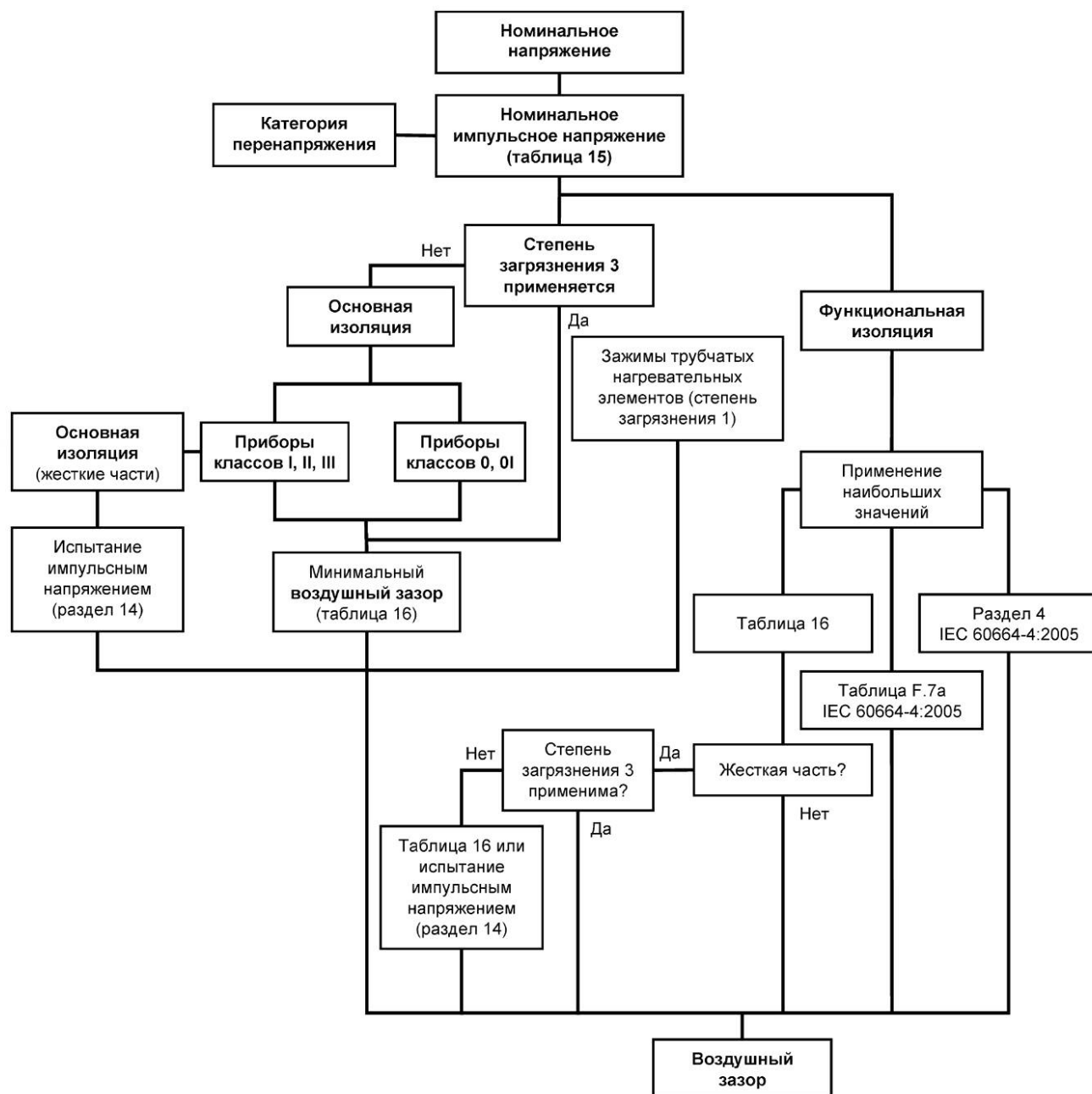
Рисунок L.1 — Алгоритм определения воздушных зазоров
