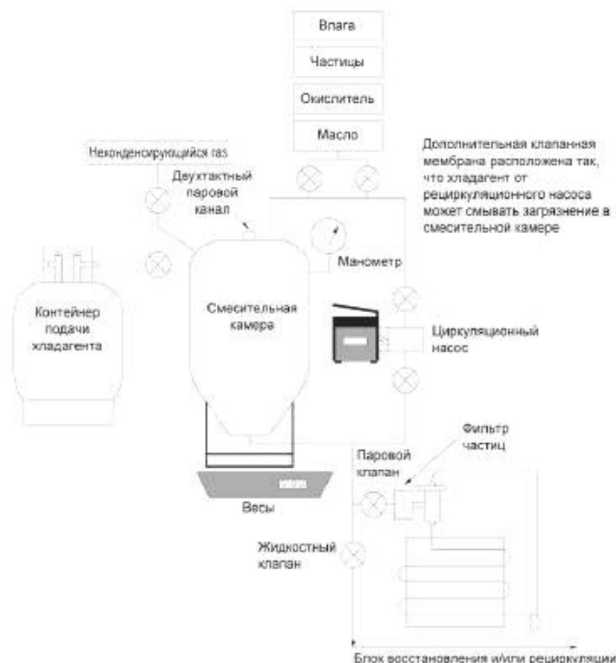
Рисунок АА.1 – Испытательная аппаратура для автономного оборудования
