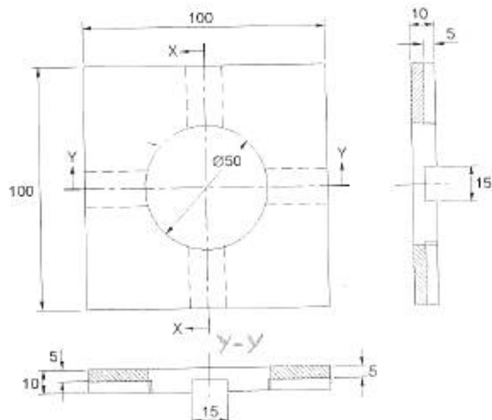
Рисунок 113а – Фрагмент А – Нижняя часть маски
