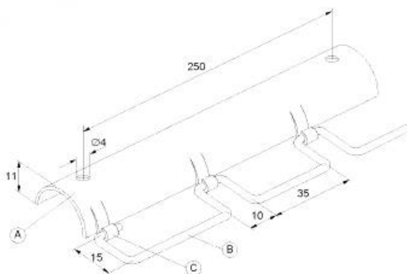
Рисунок ВВ.2 – Детальный эскиз барабана и цилиндров
