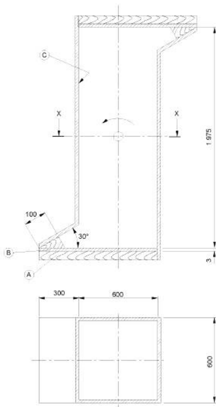
Рисунок 107 – Вращающийся барабан для испытания механической прочности подушек
