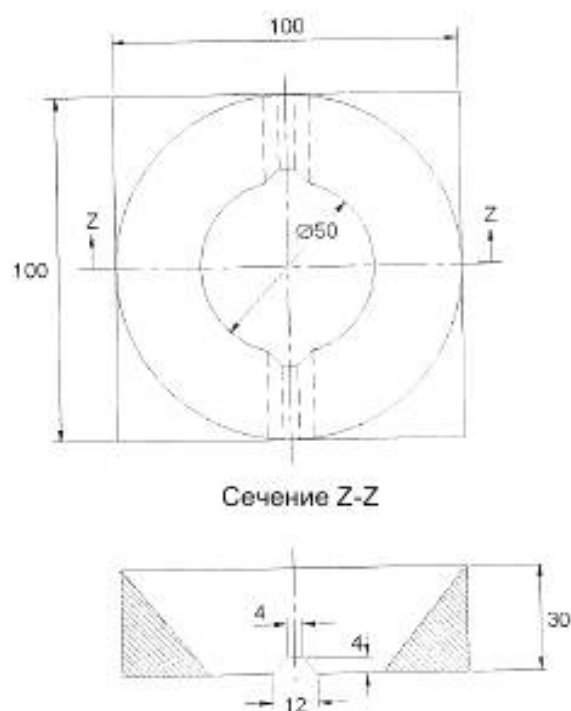
Рисунок 113б – Фрагмент В – Верхняя часть маски
