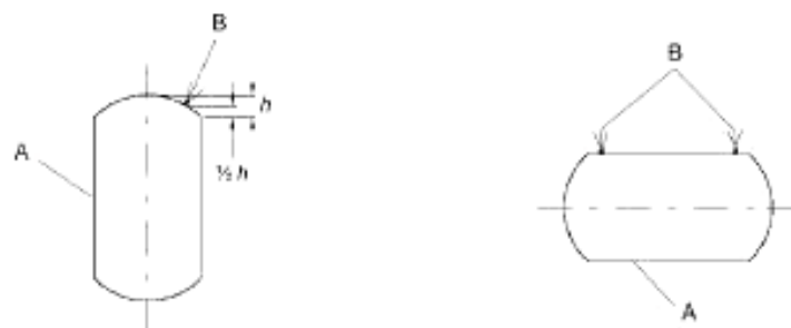
Рисунок 102 – Пример расположений термопар
