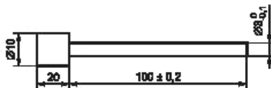
Рисунок 101— Испытательный стержень для скрытой блокировки
