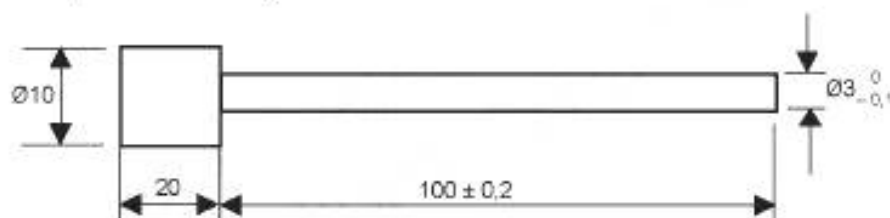
Рисунок 101 — Испытательный прут для скрытой блокировки
