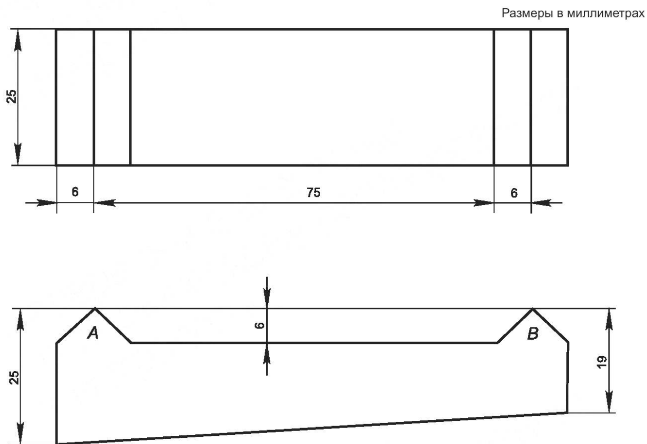
Рисунок 102 — Имитируемая рука
