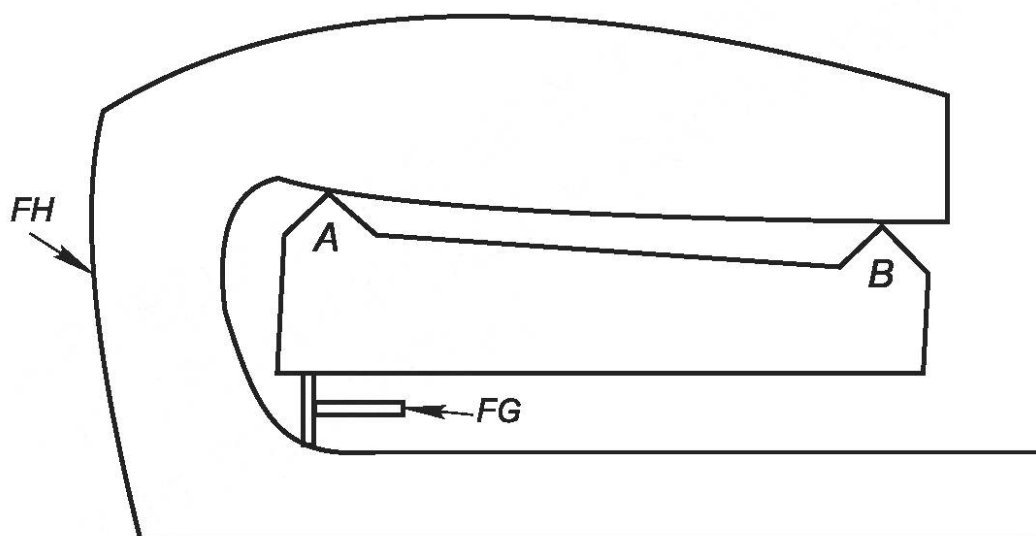
Рисунок 105 — Расположение имитируемой руки в незамкнутой рукоятке
