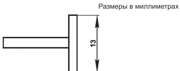
Рисунок 103 — Щуп
