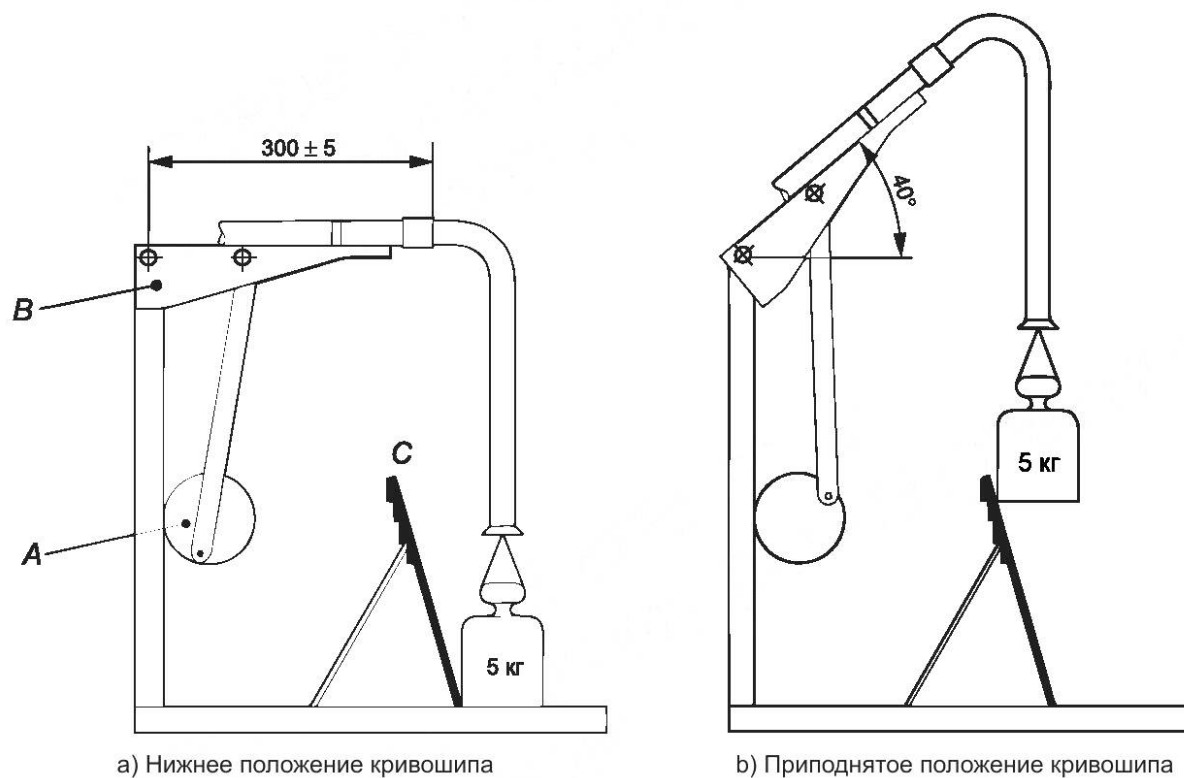
Рисунок 103 — Устройство для испытания токонесущих шлангов на перегиб
