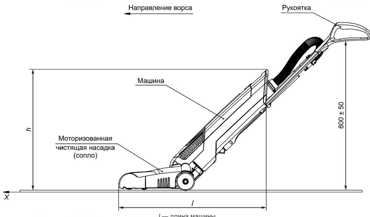
б) Машина с чистящей насадкой, оснащенная шлангом (вид сбоку)
