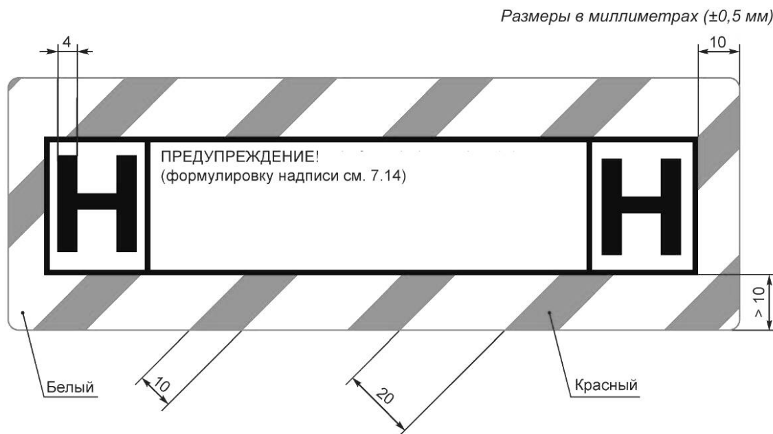
Рисунок АА.1 — Этикетка с предупреждающими символами и надписями для машин класса пыли Н
