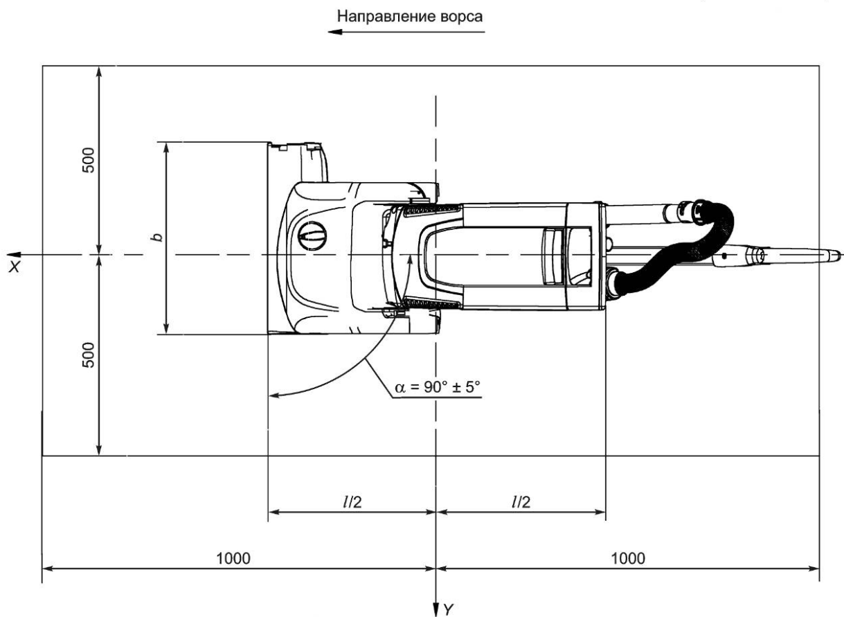
а) Машина с чистящей насадкой, оснащенная шлангом (вид сверху)
