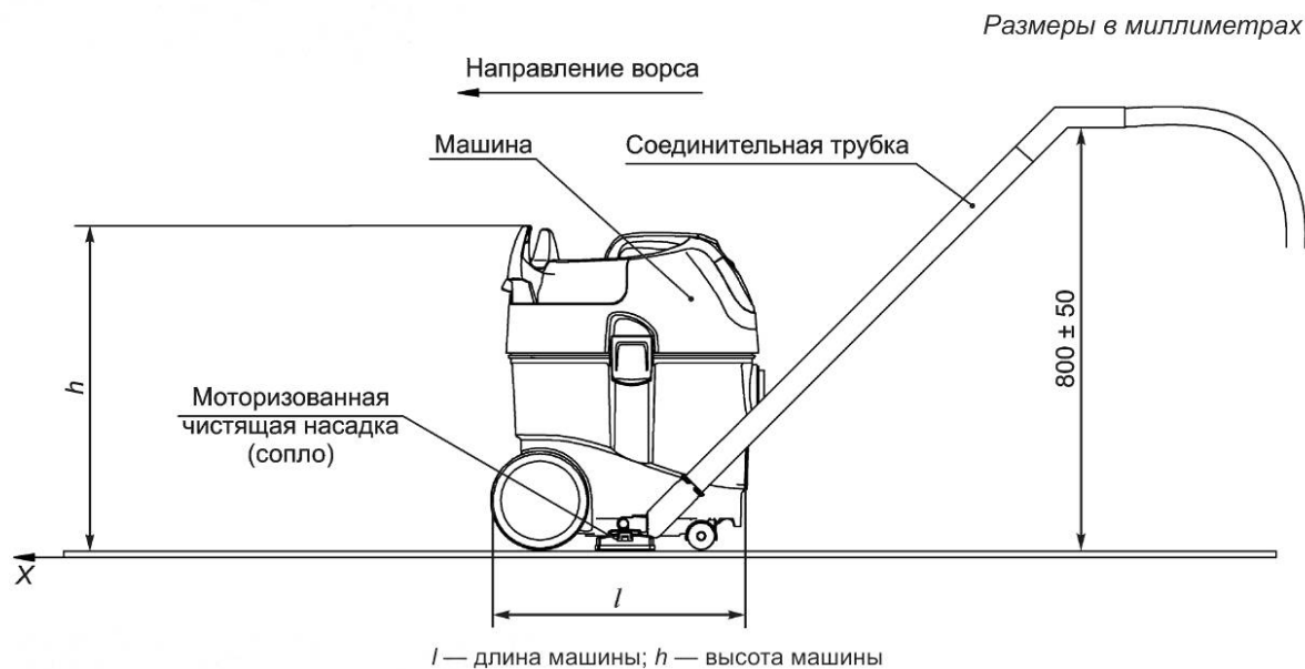
Рисунок ЕЕ.1 — Положение пылесосов и аксессуаров при испытании
