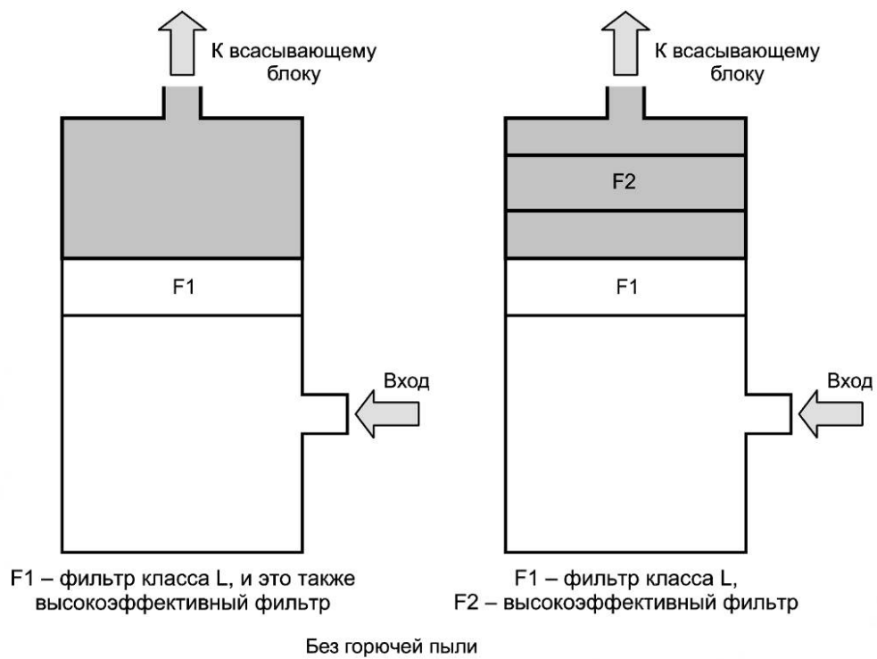
Рисунок СС.2 — Зоны, которые считаются свободными от горючей пыли
