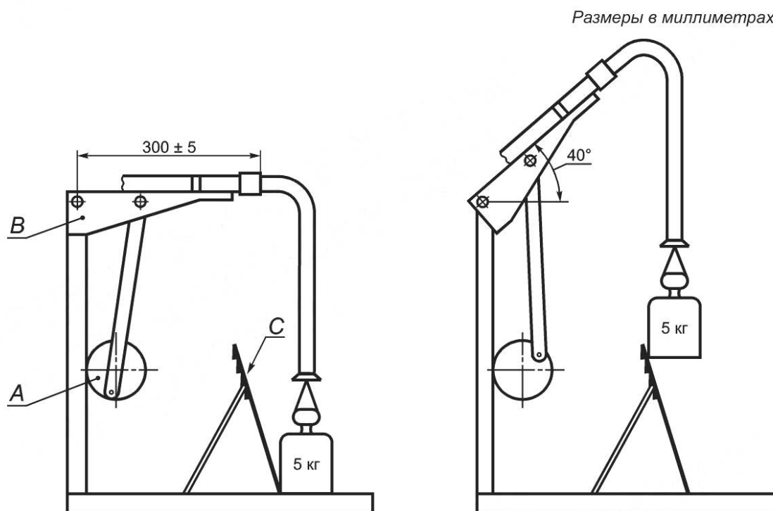
Рисунок 102 — Устройство для испытания токоведущих шлангов на истирание
