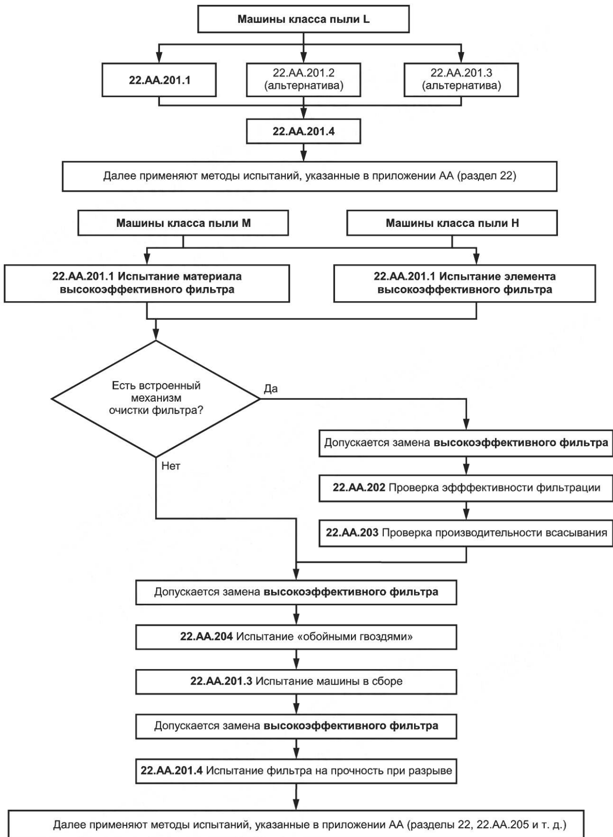
Рисунок АА.6 — Последовательность проведения и выбора испытаний, указанных в разделе 22
