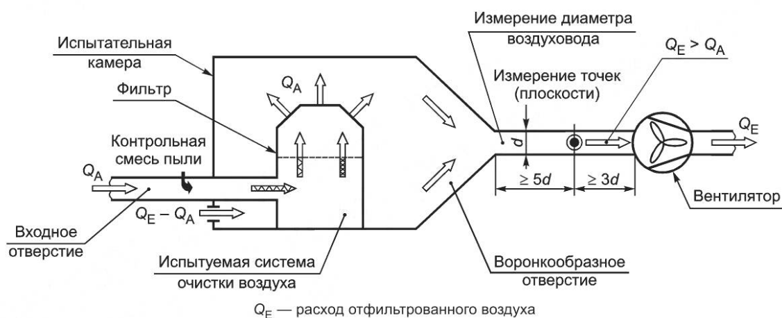
Рисунок АА.5 — Испытание системы очистки воздуха машиной
