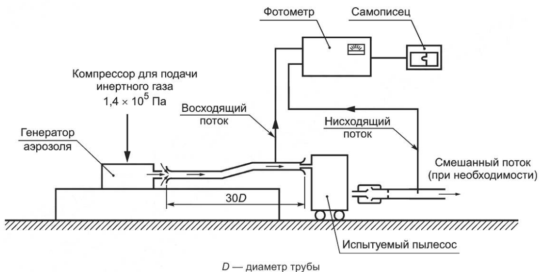
Рисунок АА.4 — Оборудование для испытания элемента высокоэффективного фильтра
