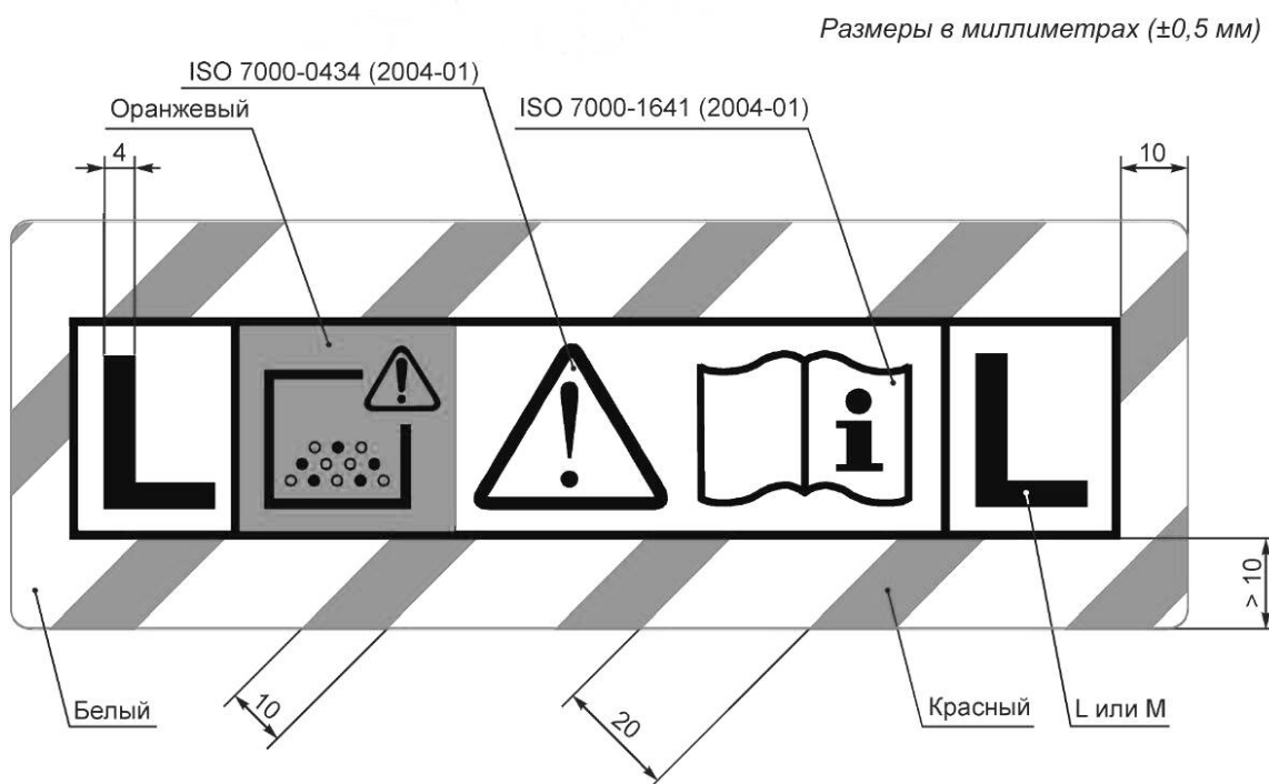
Рисунок АА.2 — Этикетка с предупреждающими символами для машин классов пыли L и M
