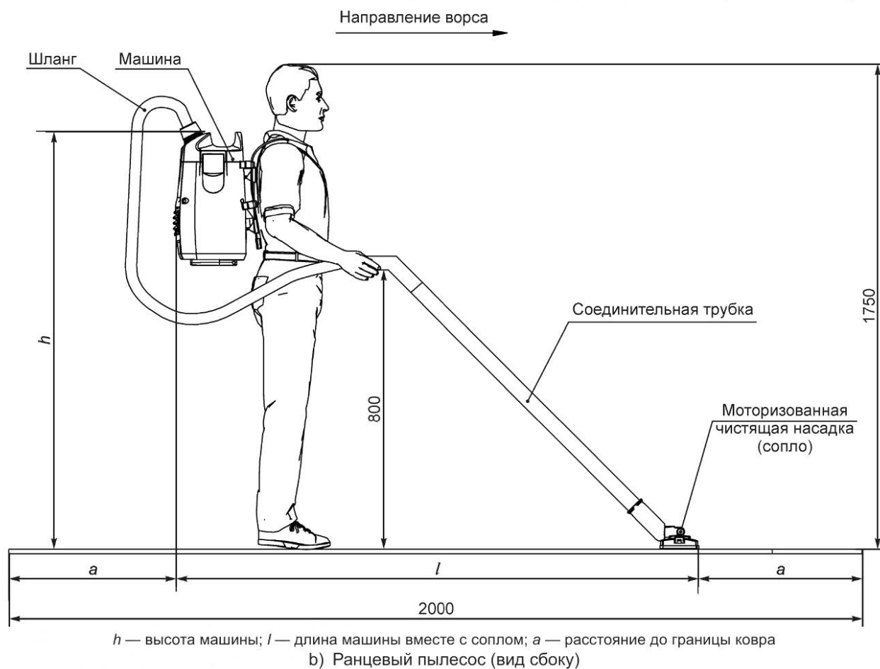
Рисунок ЕЕ.3 — Расположение рюкзаковых пылесосов
