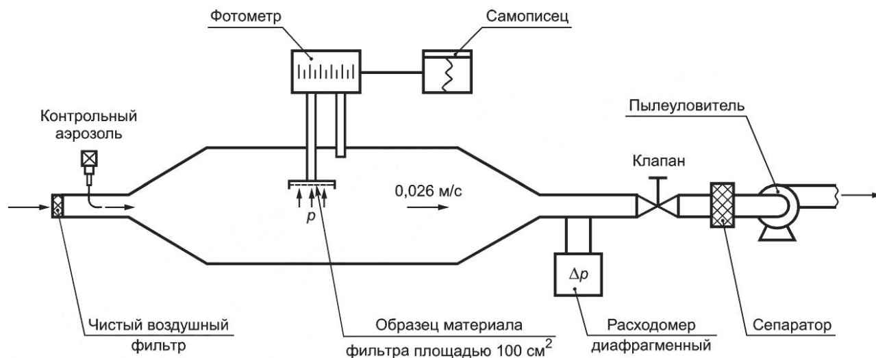
Рисунок АА.3 — Оборудование для испытания материала высокоэффективного фильтра
