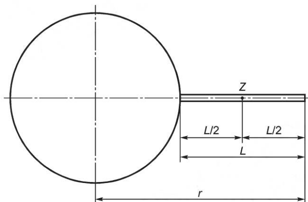
Рисунок 105а — Линия режущей нити
