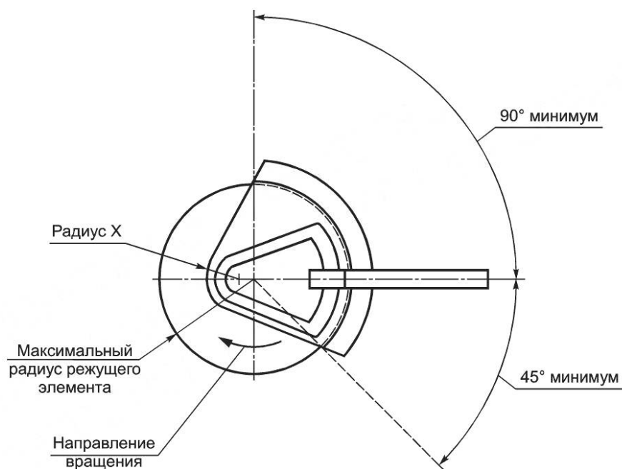
Рисунок 101a — Вид сверху
