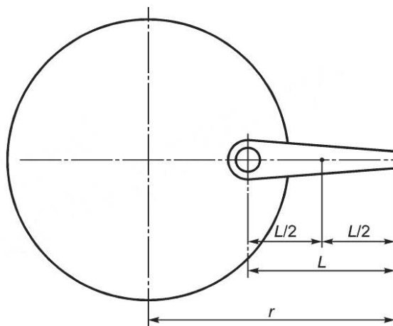
Рисунок 105b — Вращающийся режущий элемент
