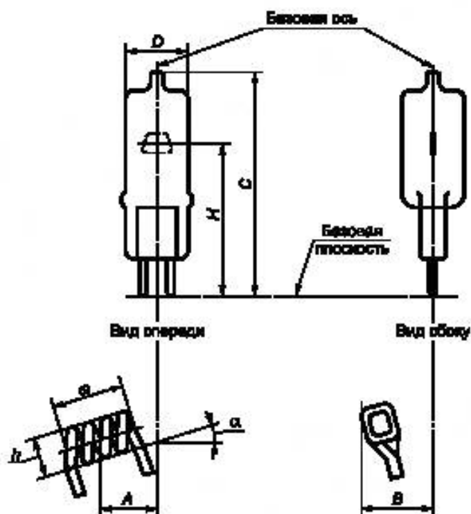
Совмещенные диаграммы лампы и тела накала
