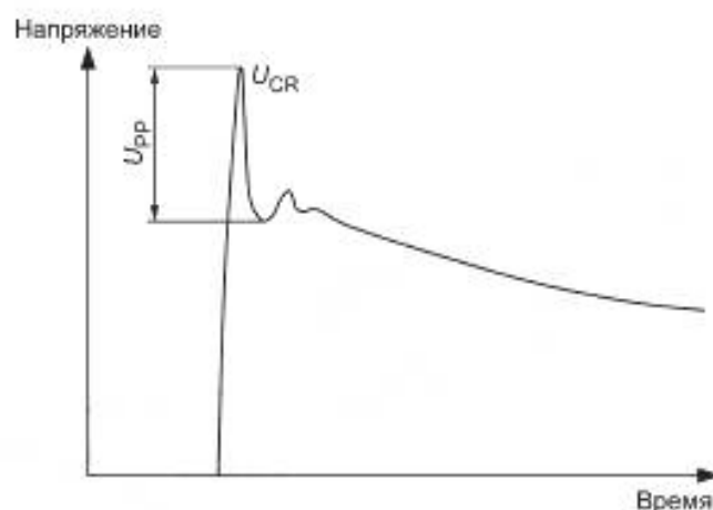
Рисунок 7 — Форма импульсной волны
