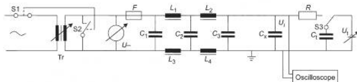
Рисунок 8 — Типовая схема для импульсной нагрузки испытуемых конденсаторов
