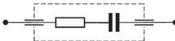
Рисунок 2 — Резисторно-конденсаторное звено
