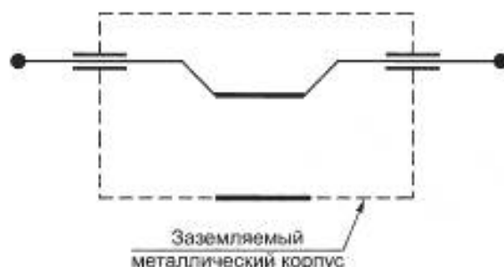
Рисунок 4b — Проходной конденсатор для асимметричного использования (некоаксиальный)
