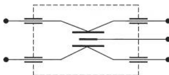
Рисунок 4d — Многозвенный проходной конденсатор
