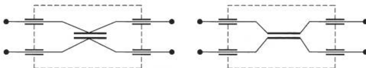
Рисунок 4а — Проходной конденсатор для симметричного использования (некоаксиальный)
