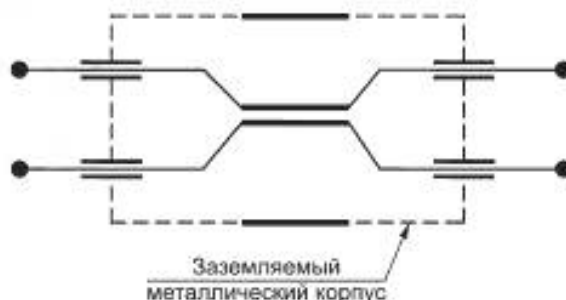
Рисунок 4c — Многозвенный проходной конденсатор (некоаксиальный) для симметричного и несимметричного использования
