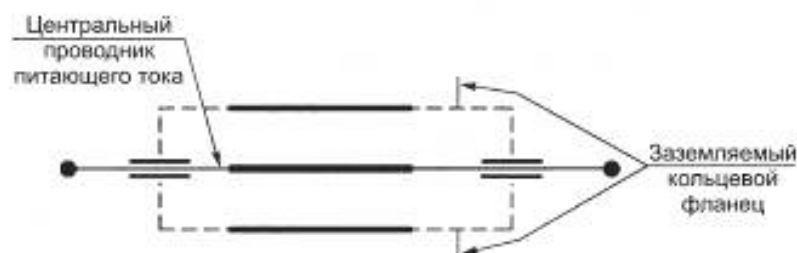
Рисунок 3 — Коаксиальный проходной конденсатор
