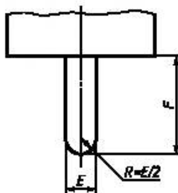
Рисунок 18 — Испытательный цоколь для испытания патронов Fa8 по разделу 13
