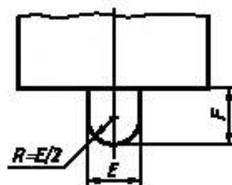
Рисунок 20 — Испытательный цокль для испытания патронов Fa8 по разделу 13
