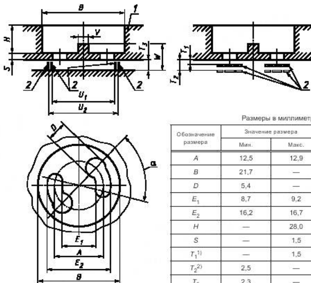
Вариант расположения контактов
