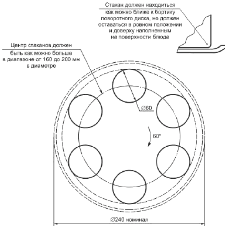
Рисунок 1 — Расположение стаканов на поворотном диске микроволновой печи
